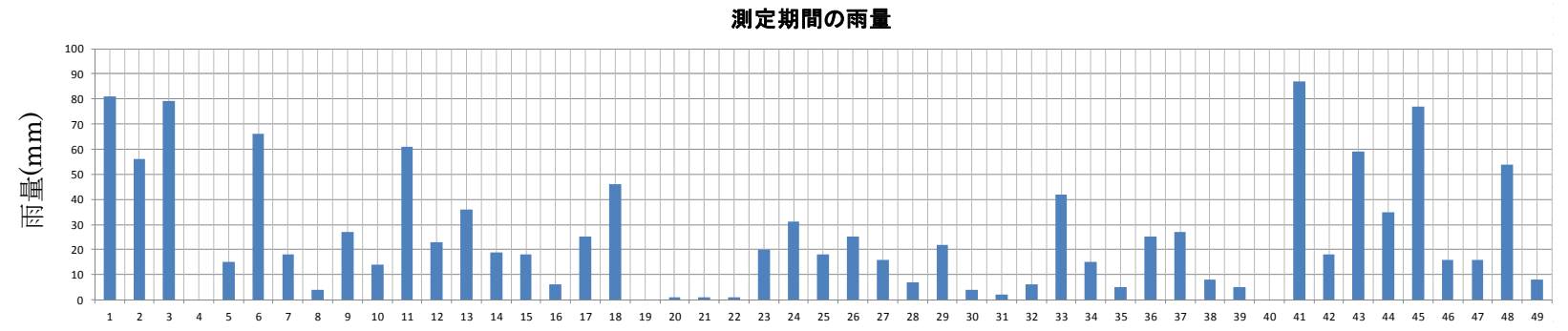
図 4.3.1 法面観測データ平成 22 年 7 月～平成 23 年 7 月
