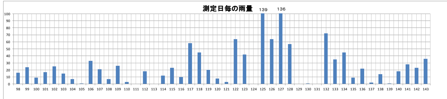
図 4.3.3 法面観測データ平成 24 年 11 月～平成 25 年 12 月
