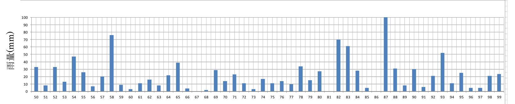
図 4.3.2 法面観測データ平成 23 年 7 月～平成 24 年 11 月
