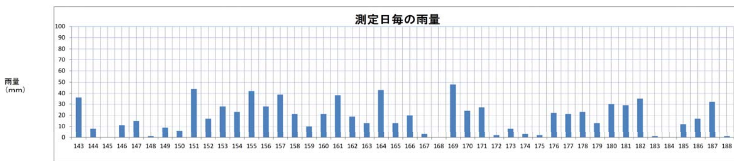
図 4.3.4 法面観測データ平成 27 年 4 月～平成 27 年 5 月
