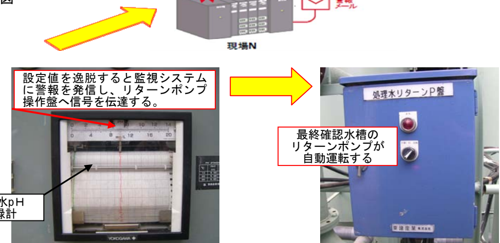
図 5.3.2 排出基準逸脱時の警報・自動返送機能
