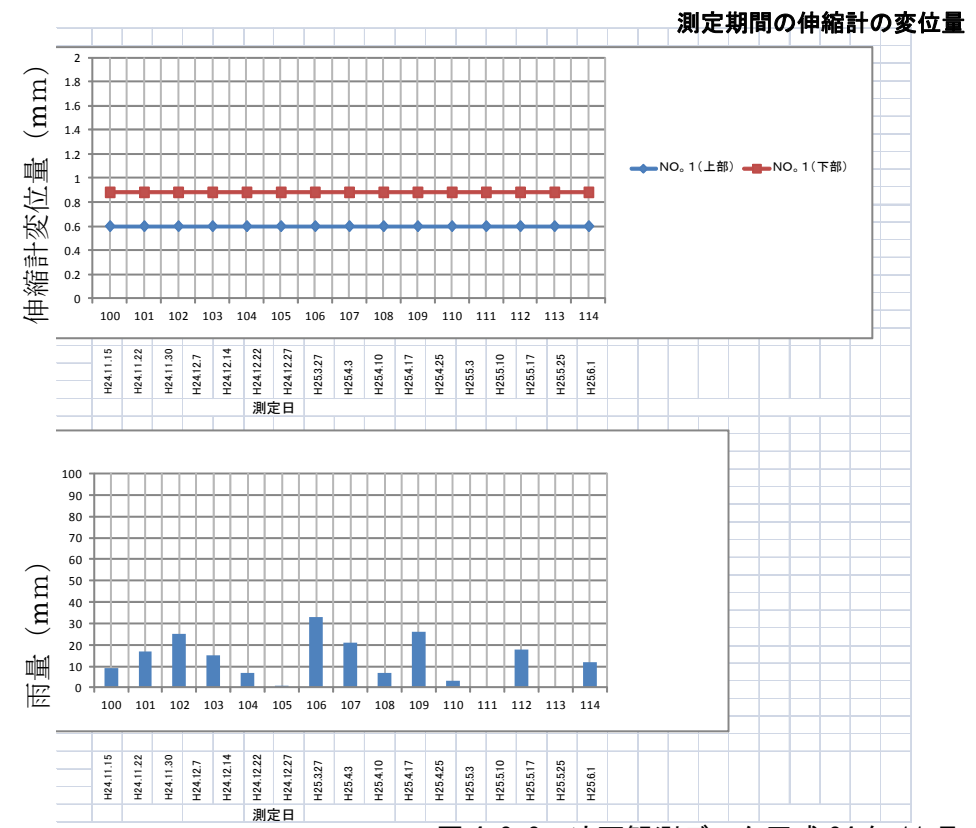
図 4.3.3 法面観測データ平成 24 年 11 月～平成 25 年 6 月
