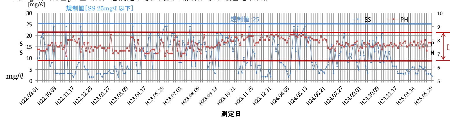
図 5.3.1 濁水処理後の放流水
