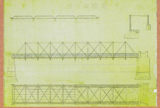
長野県初の洋式道路橋・上田橋設計図（複製）（明治23年、当館蔵）
