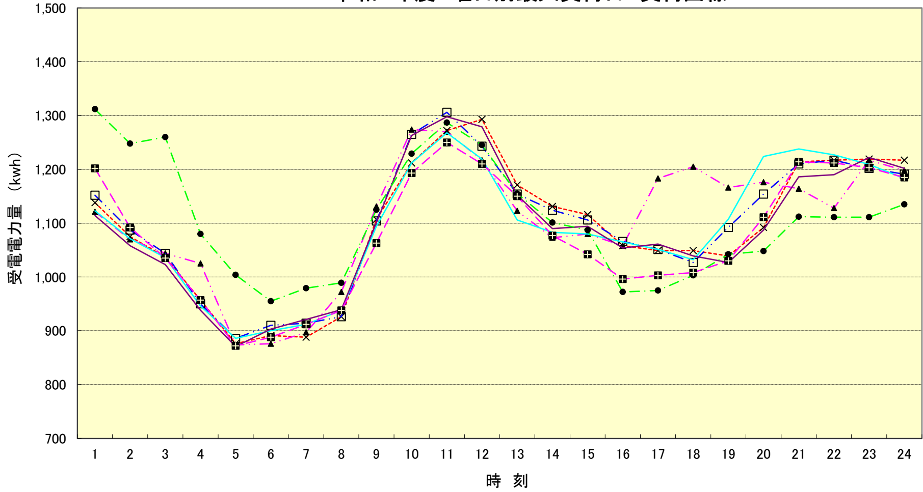
令和4年度 曜日別最大負荷日 負荷曲線
