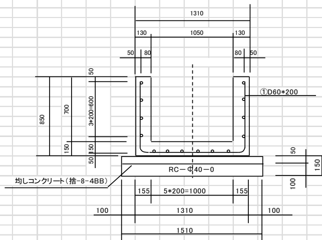
標準断面図
