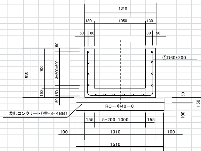
標準断面図
