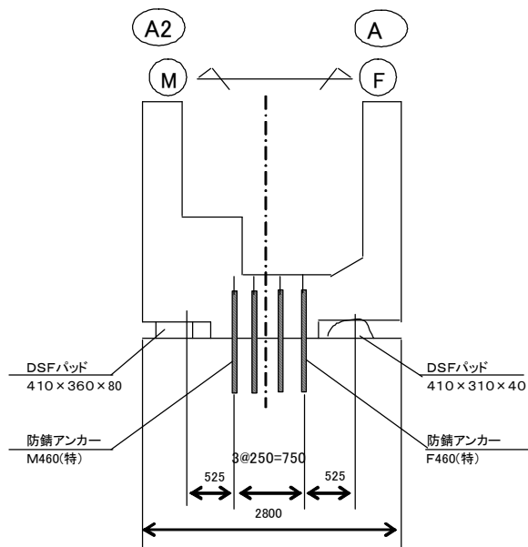
断面図 S = 1 : 40
