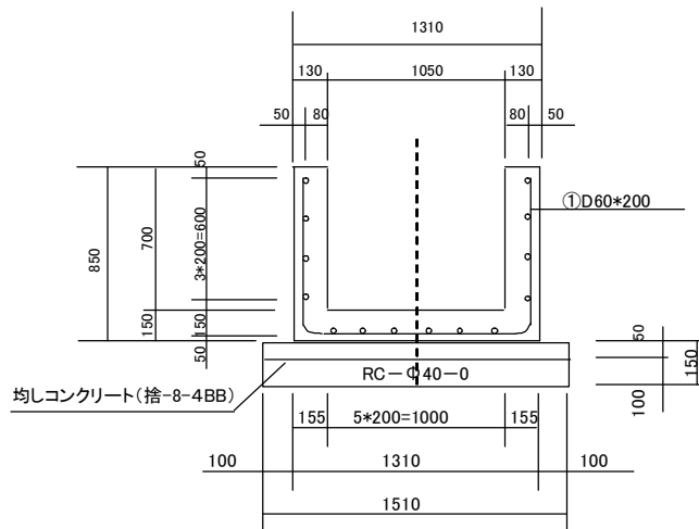
標準断面図
