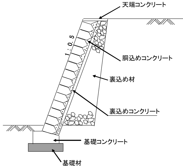
標準断面図
