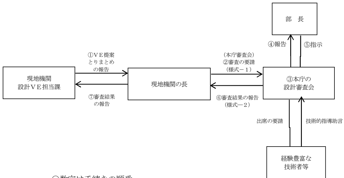
別図－３ (3) 設計VE審査手続
