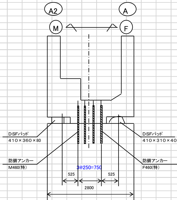
断面図 S = 1 : 40
