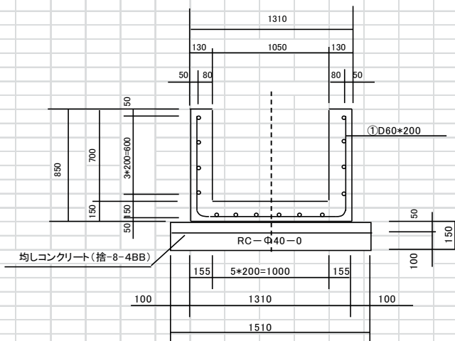
標準断面図
