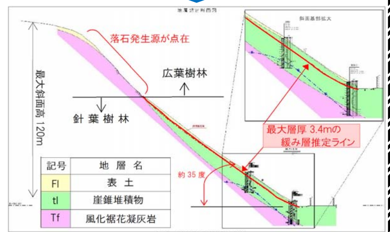
図 地層想定断面図
