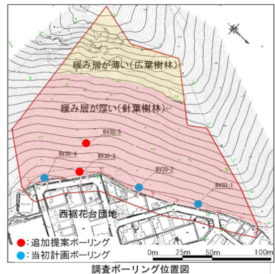
調査ボーリング位置図
