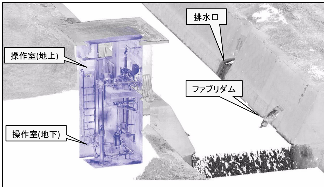
【ファブリダム位置の取水施設の断面】
