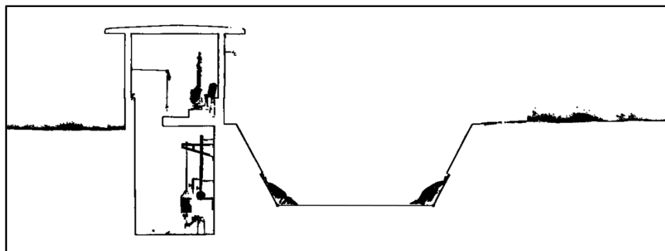
【ファブリダム位置の取水施設の断面】
