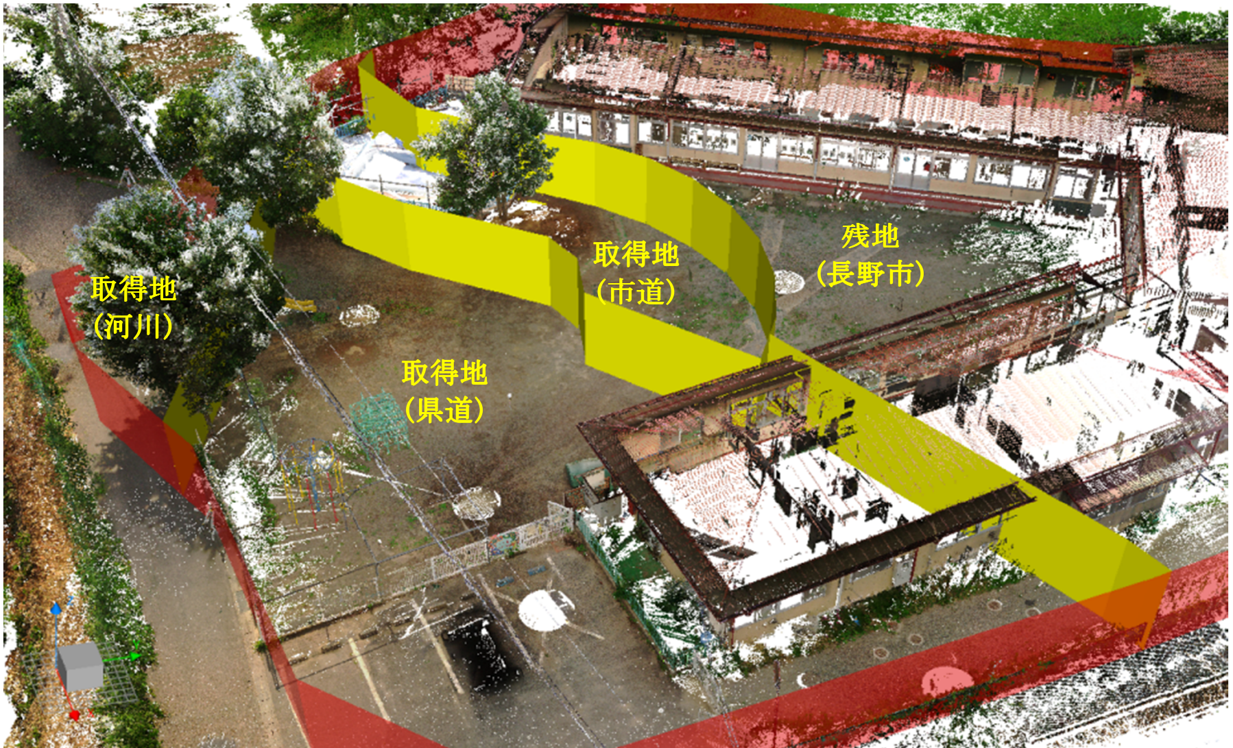
〈地上型レーザスキャナによる点群データをのせた境界説明図面〉 赤線：境界線、黄線：取得線
