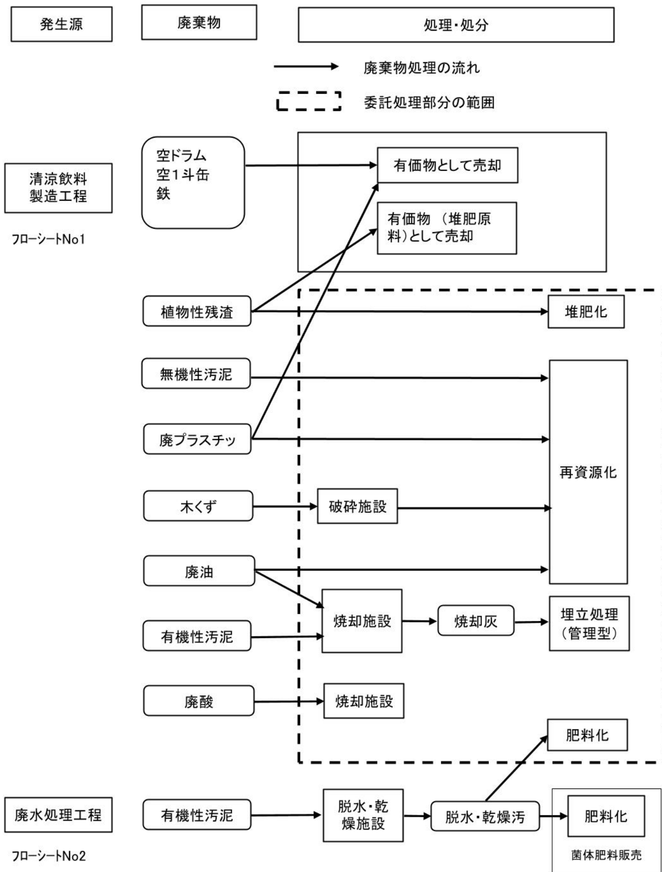
図3 廃棄物処理フロー図（現状）
