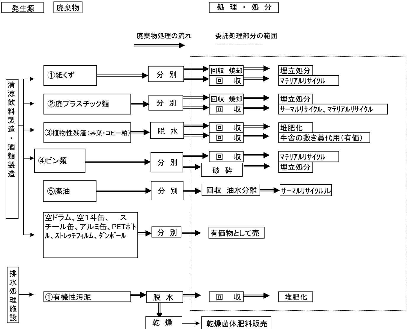
図3 廃棄物処理フロー図
