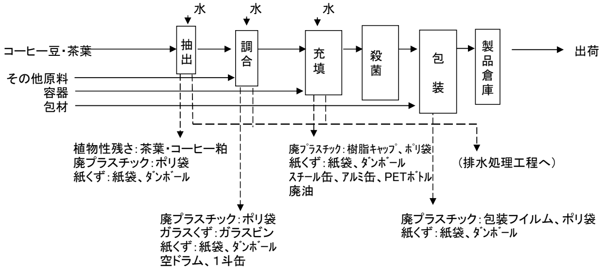
図1 清涼飲料・酒類製造フローシート
