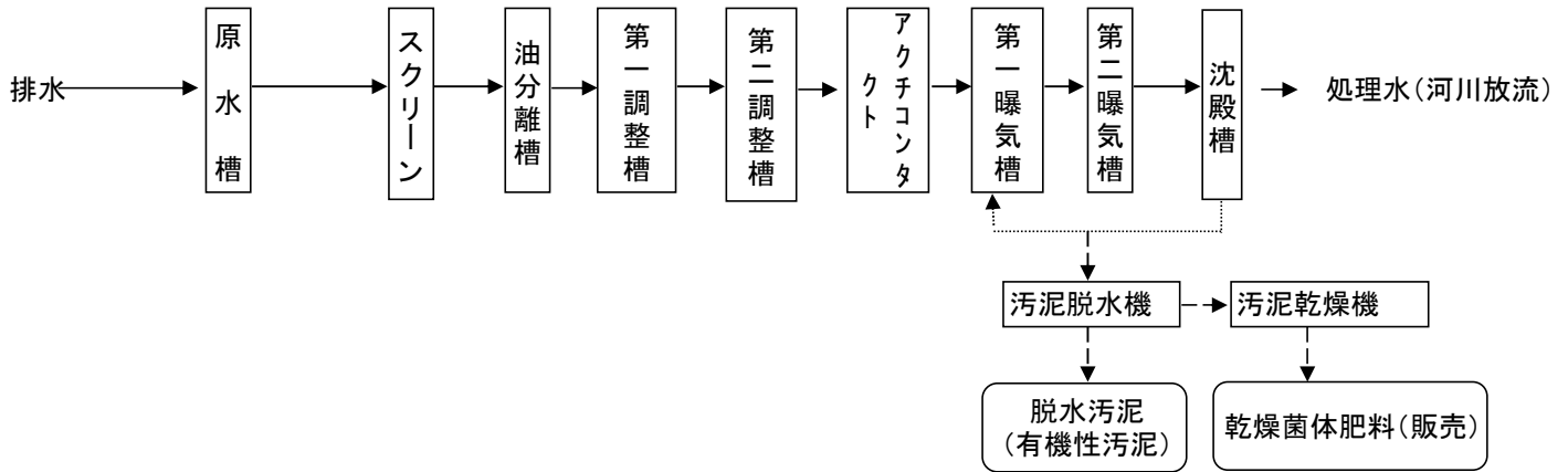
図2 排水処理フローシート
