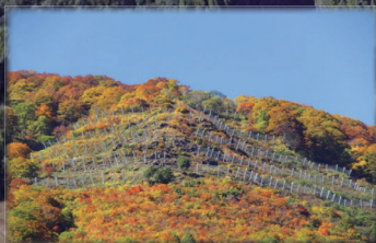
白馬村 飯田 雪崩防止柵
