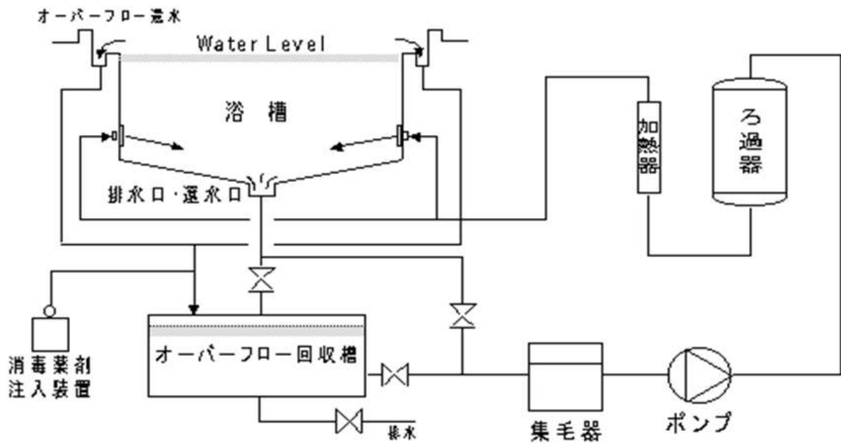
図-3 側壁吐出・オーバーフロー還水方式
