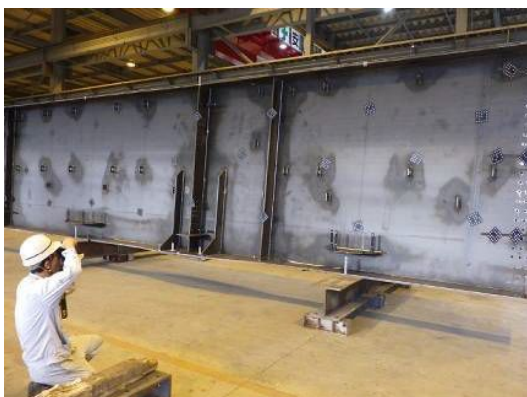
橋桁 出来形測定(カメラ計測)
