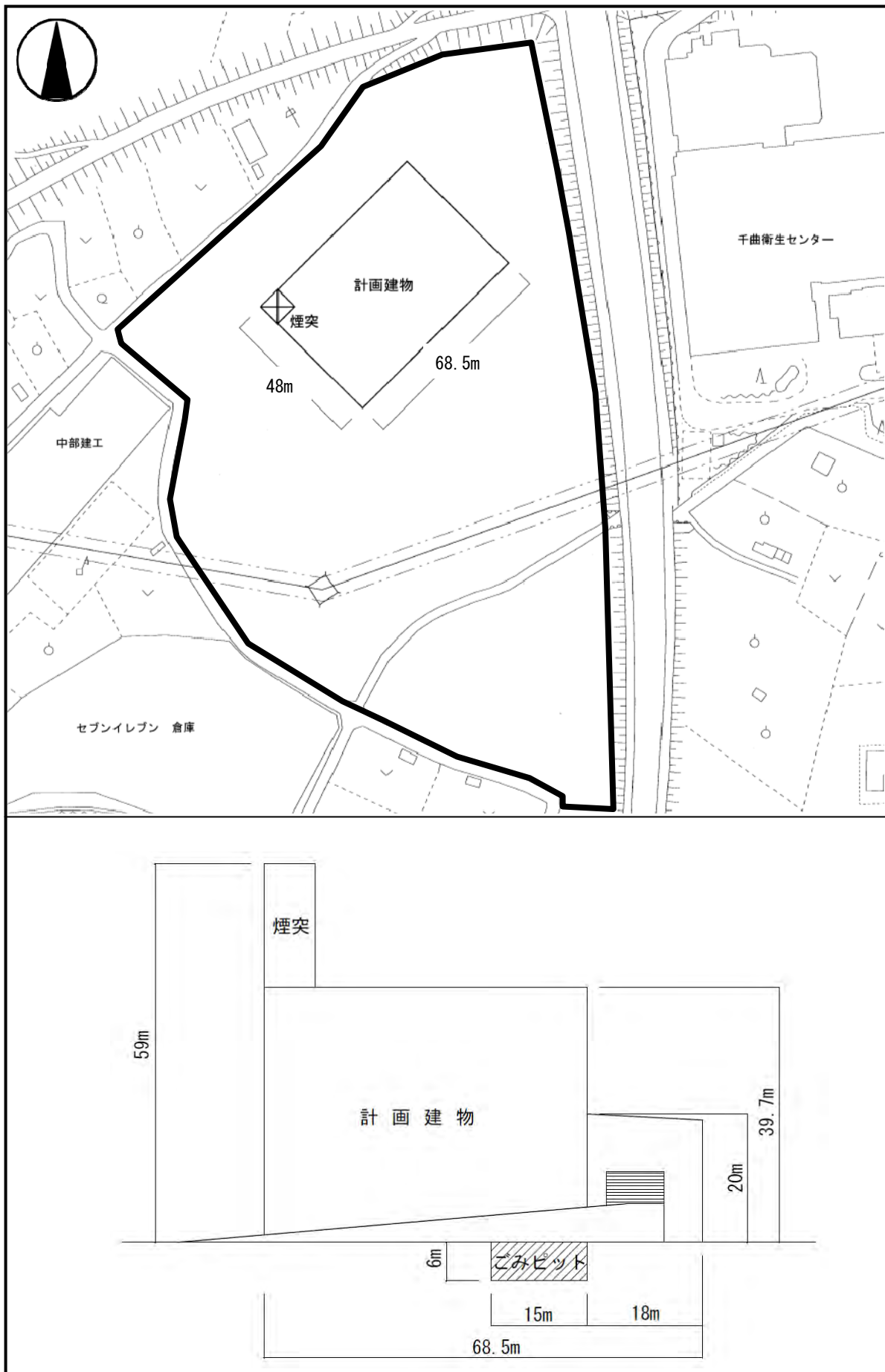
図 1-7-3(2) 全体配置計画図 (案)、断面図 (案) 【流動床式ガス化溶融方式】
