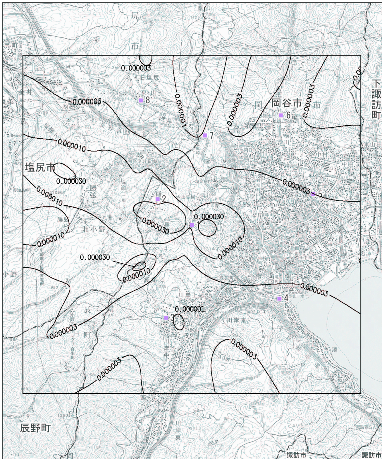
図 4-1-6 (1) 二酸化硫黄濃度分布予測結果 (年平均寄与濃度、地上)
