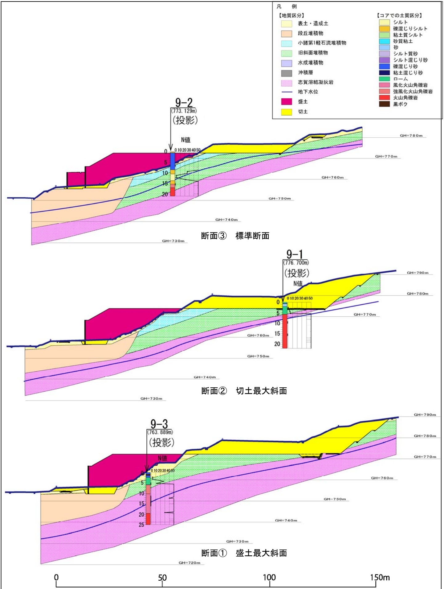
図 5-10-14(2) 造成断面図
