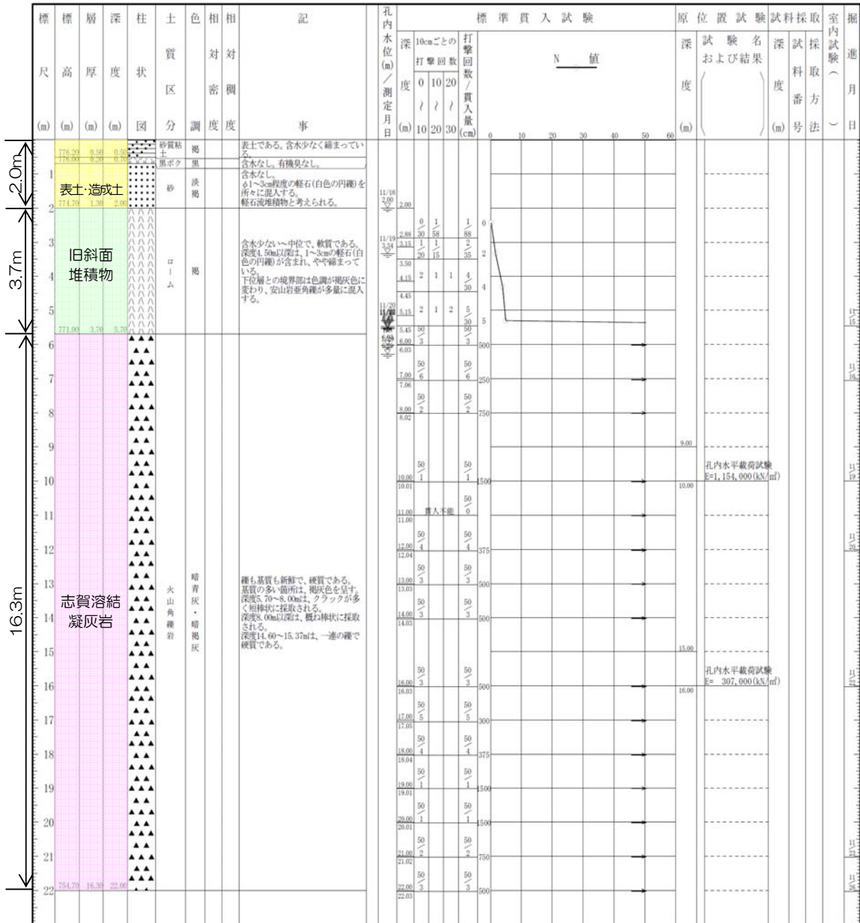
図5-10-9(1) ボーリング柱状図
