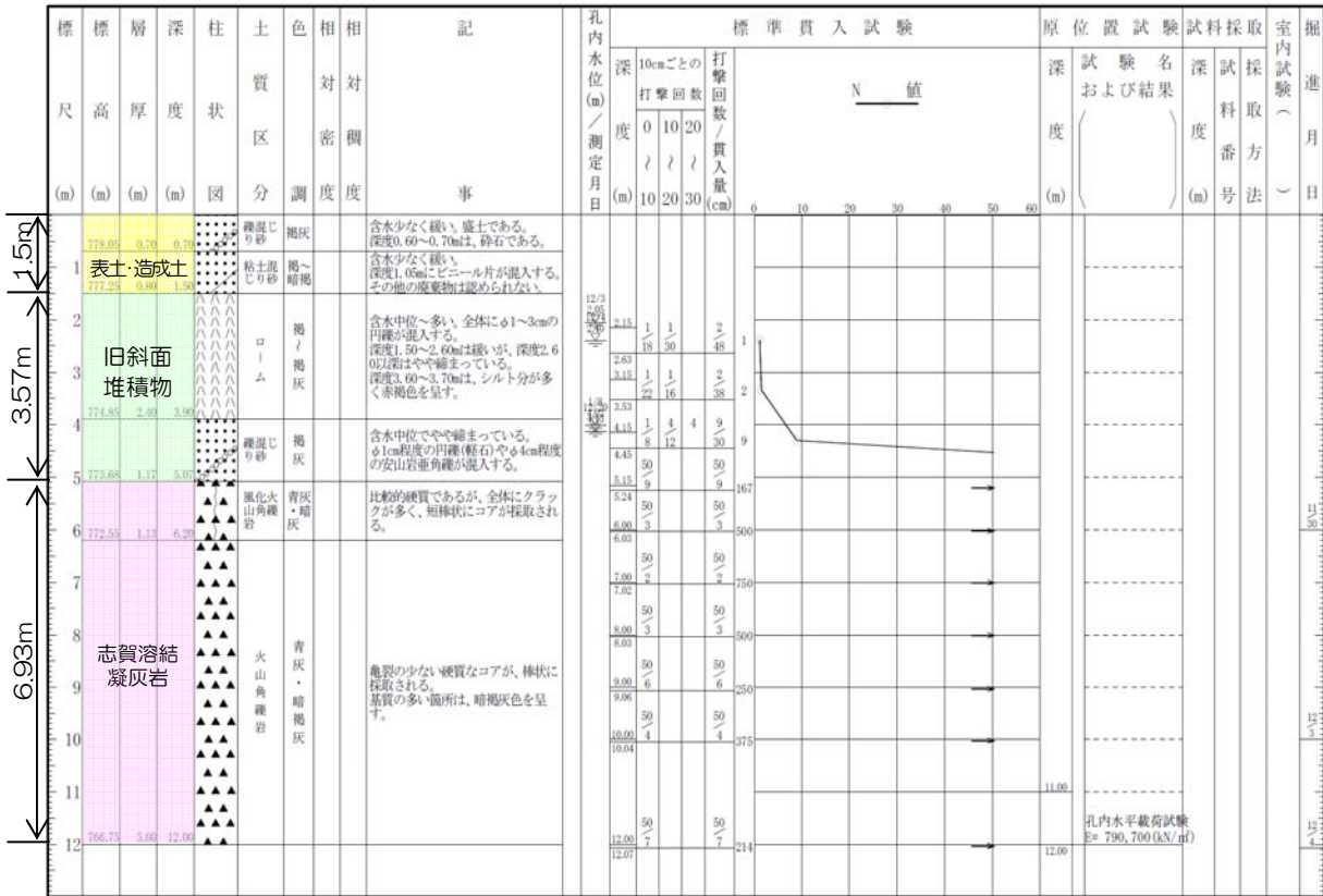
図5-10-9(6) ボーリング柱状図
