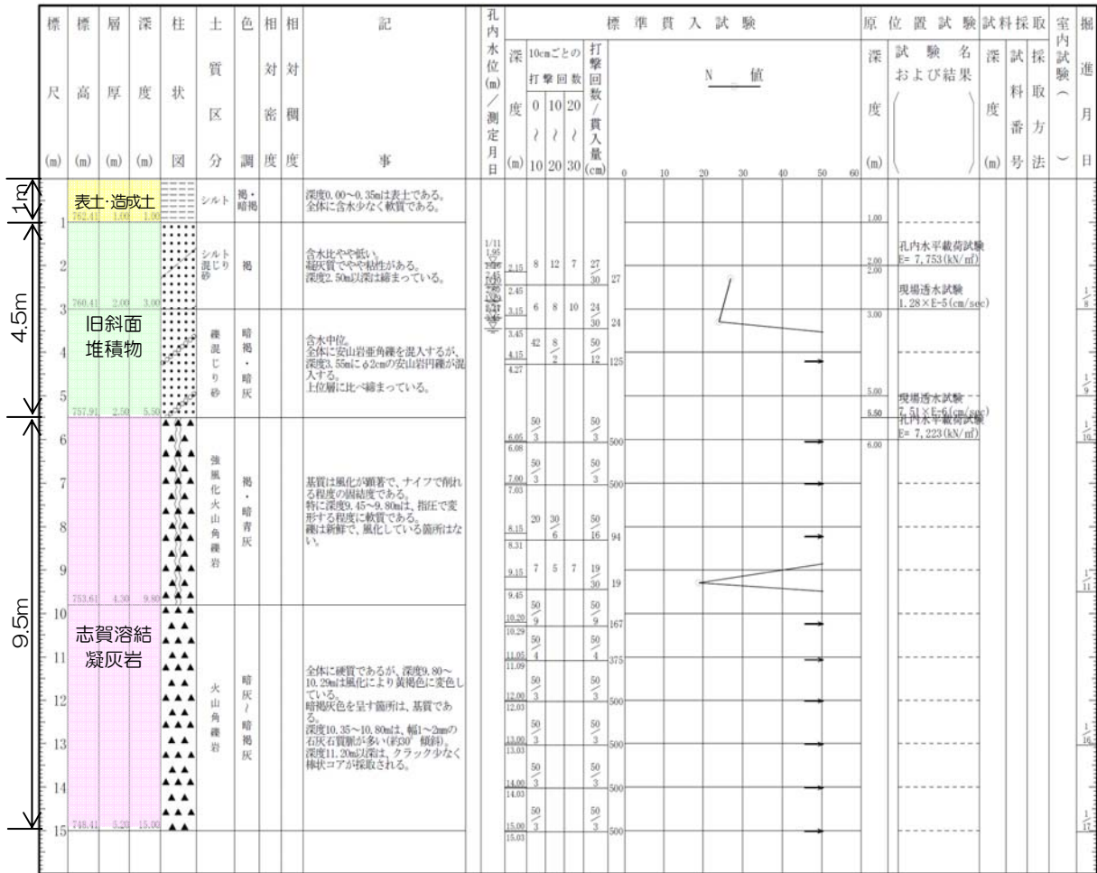
図5-10-9(4) ボーリング柱状図
