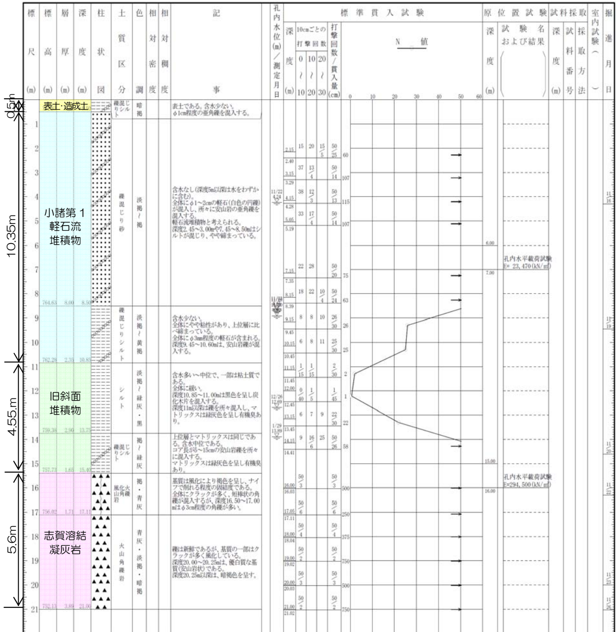
図5-10-9(2) ボーリング柱状図
