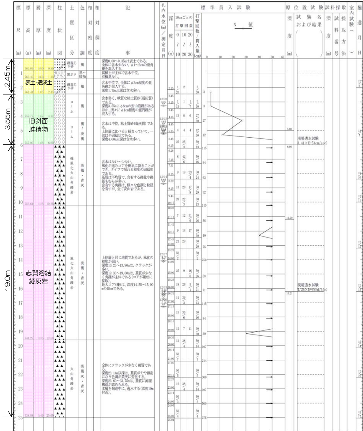
図5-10-9(3) ボーリング柱状図
