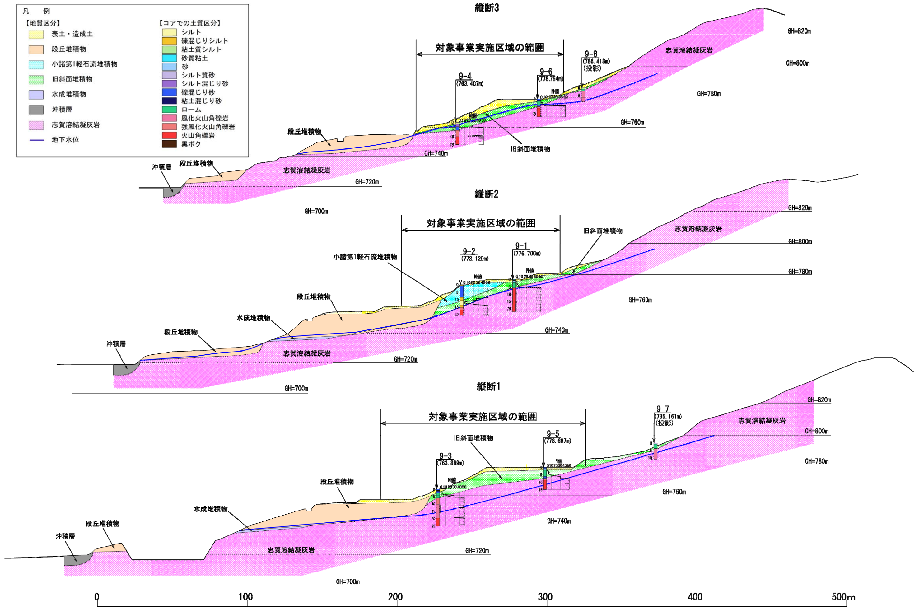
図 5-10-7 地質縦断図
