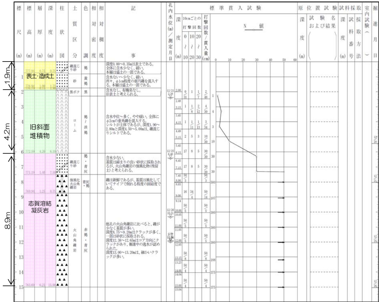
図5-10-9 (5) ボーリング柱状図
