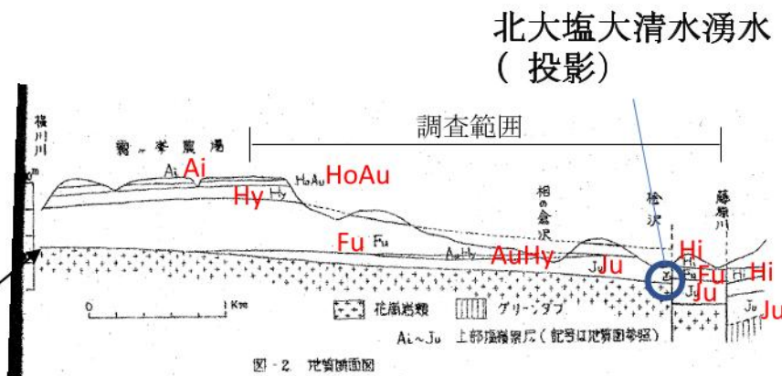
図-2 地質断面図
