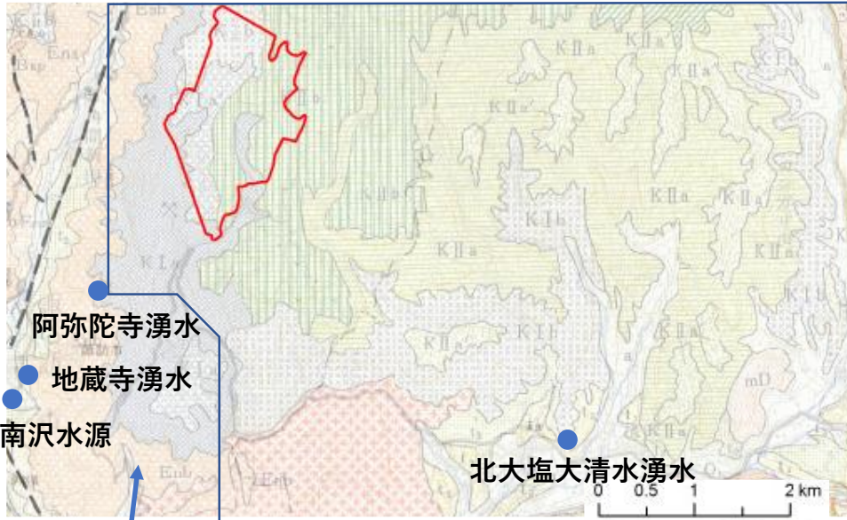
【諏訪の自然誌・地質編編集委員会(1975)の地質図】
