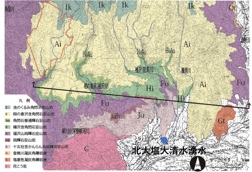
【熊井(1975)の地質図】
