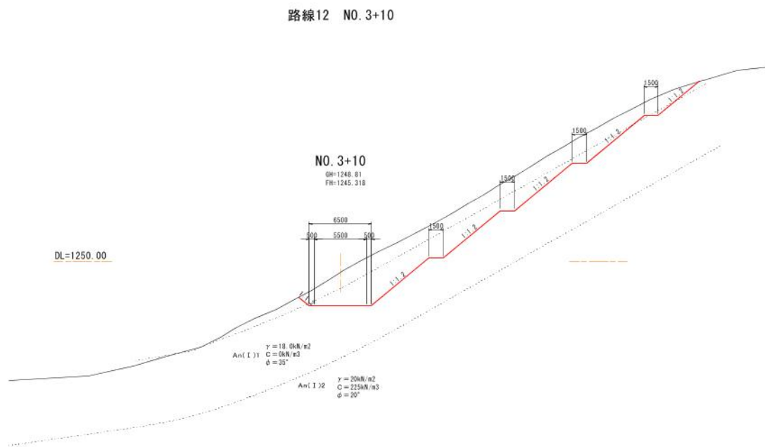
図 1-2 切土法面検討断面図
