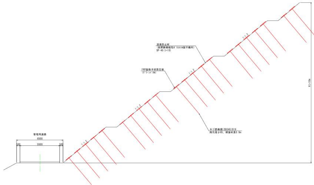
図 1-3 切土法面工
