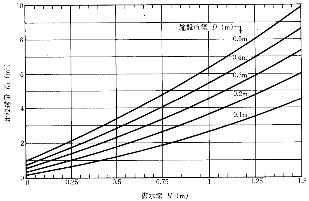
図 3-6 ポアホール法の比浸透量
