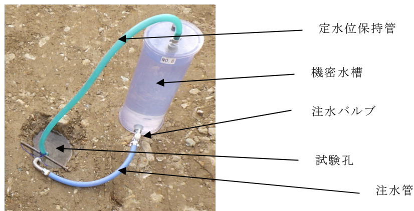
図 3-8 マリオットサイフォンを用いた試験施設 (例)
