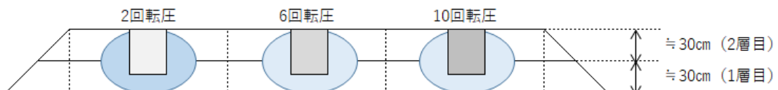
図 3-2 透水係数試験の概念断面図
