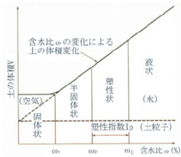
図 2-3 土のコンシステンシー限界
