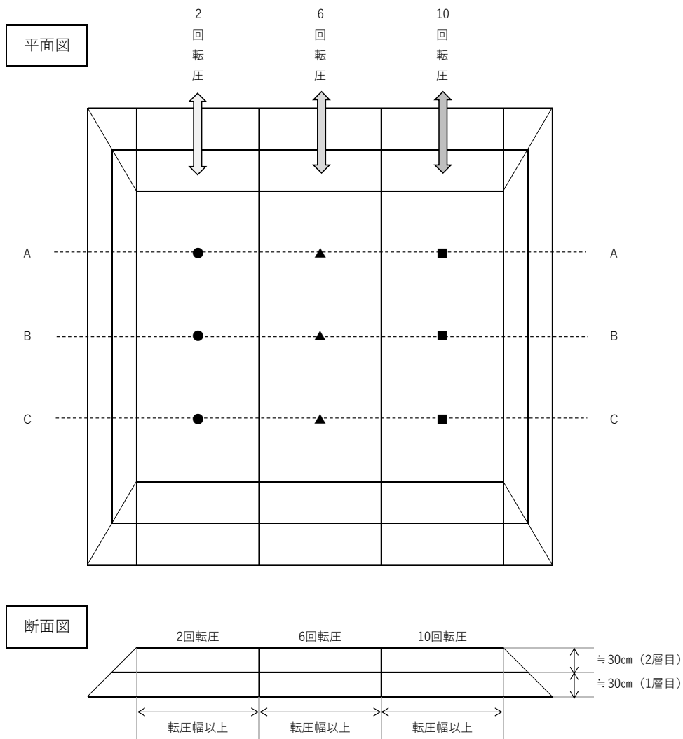
図 3-1 試験ヤード
