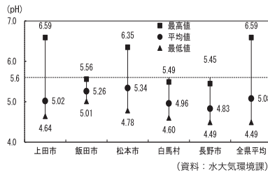
図2-4-29 酸性雨調査結果
