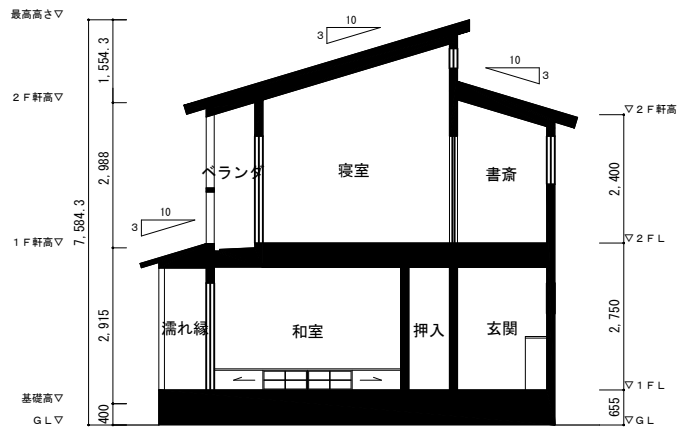
断面図 (B-B')
