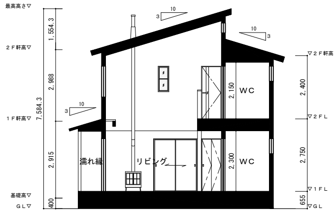
断面図 (A-A')
