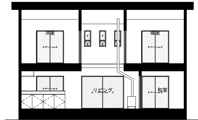
断面図 (D-D')
