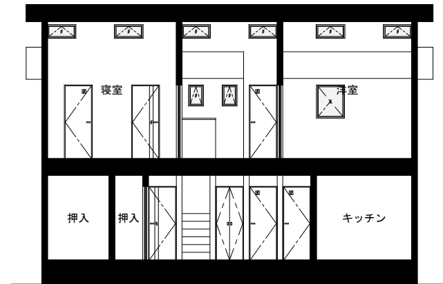
断面図 (C-C')
