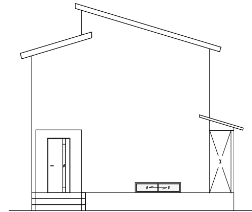
西立面图
