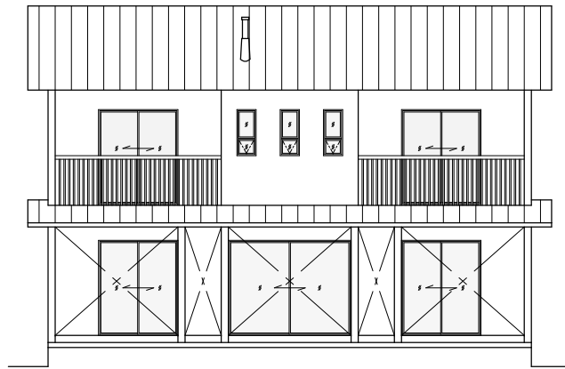
南立面图
