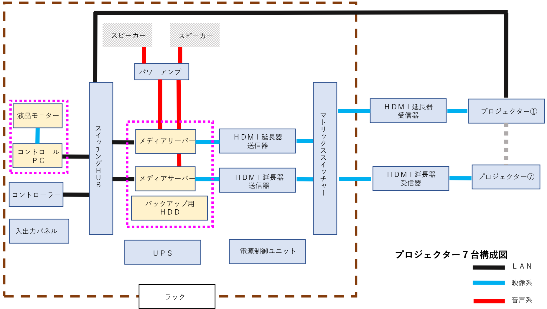
システム全体構成図 (概要)
