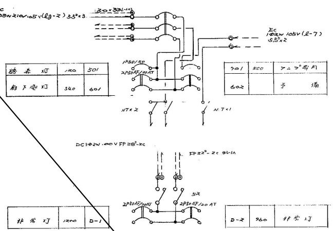
2L-1 電灯分電盤配線図
