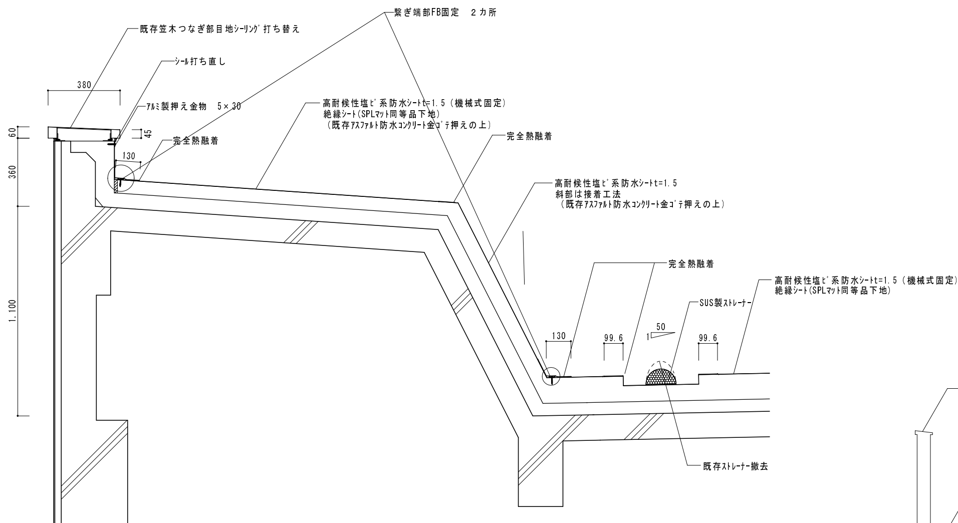
1通り側ハ'ラハ'ット納め詳細図 S=1/10
