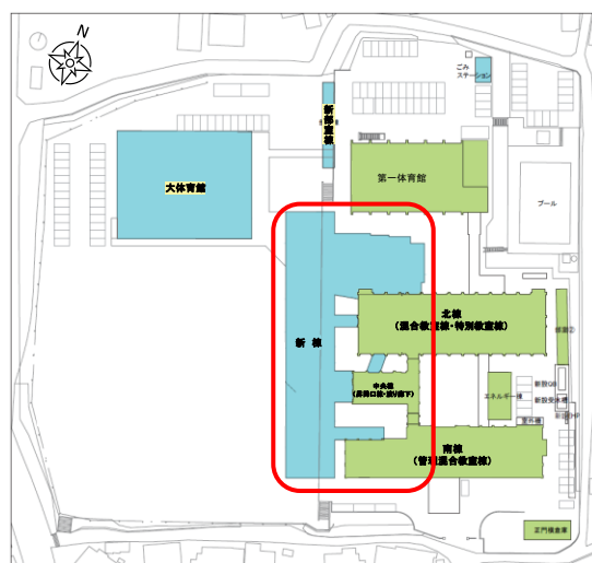
整備配置図
