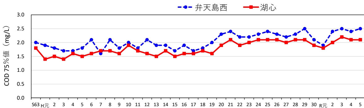
図 4 COD 75%値の推移（全層）
