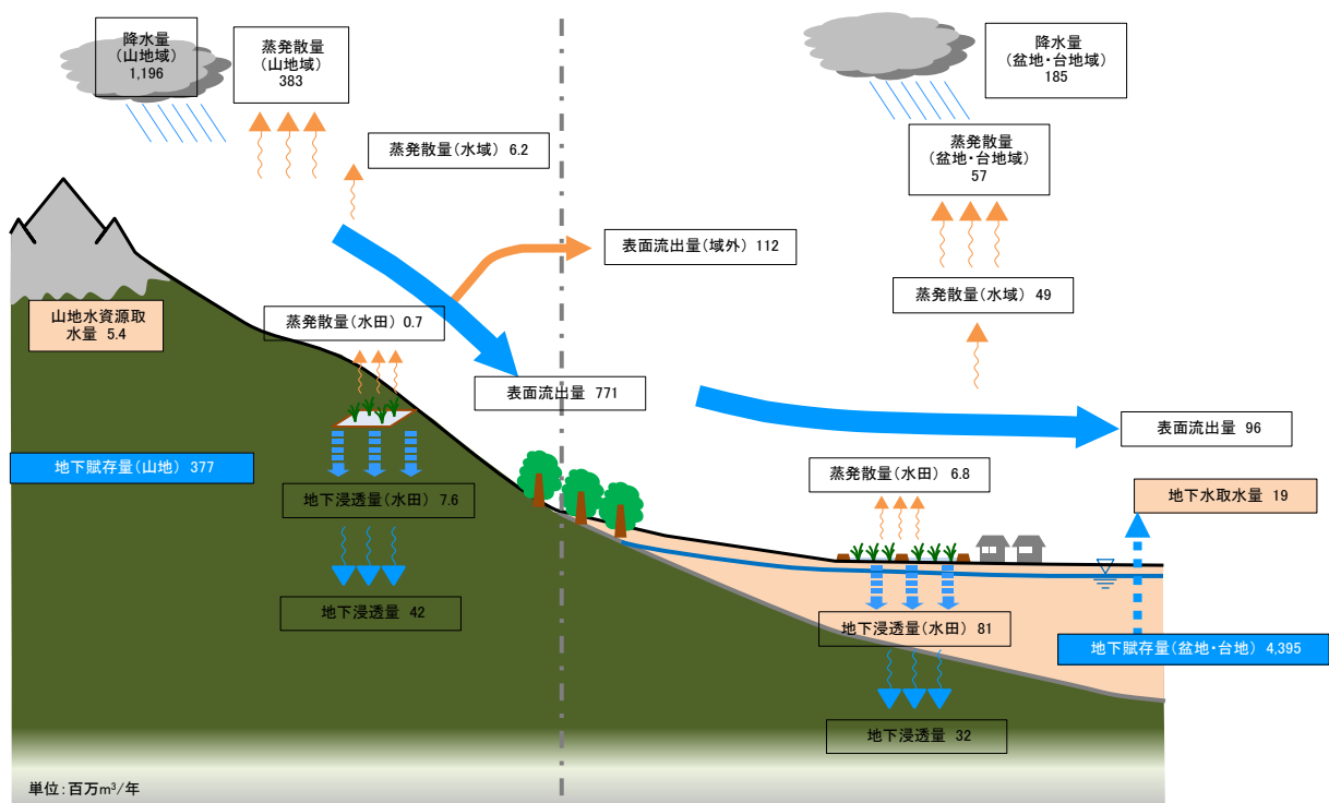
現況の水収支の模式図（大北（千曲川水系））
