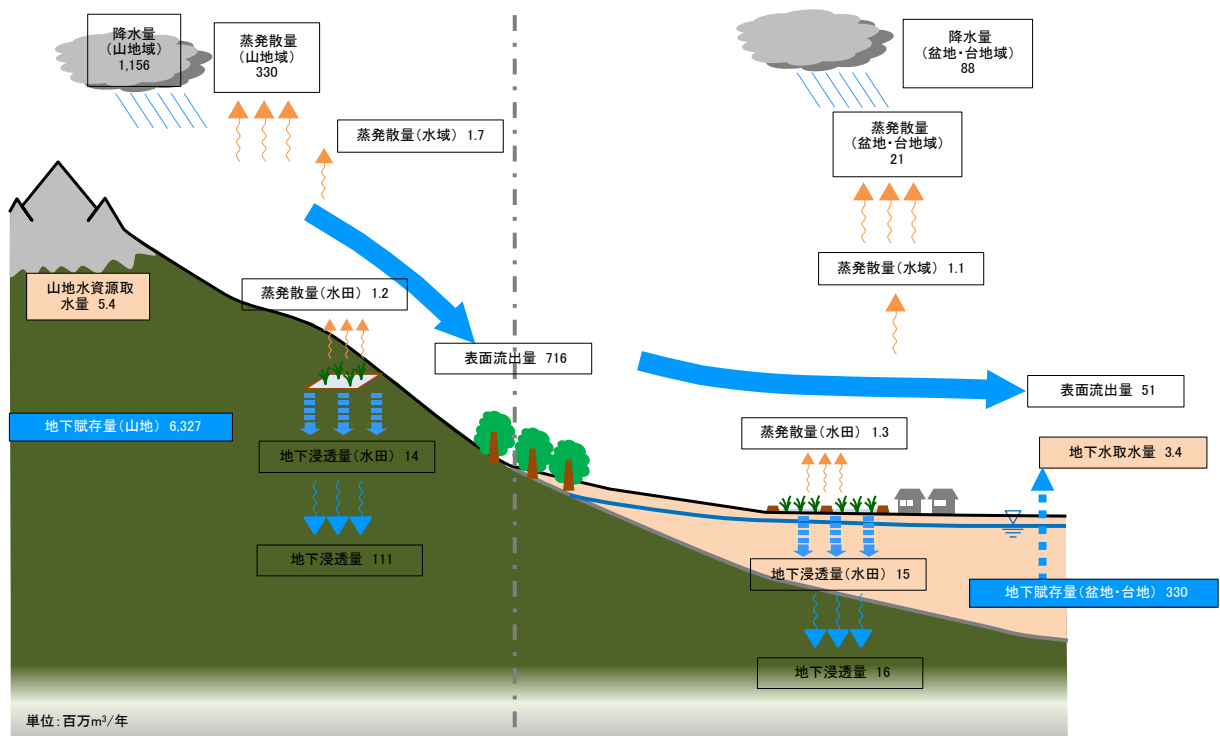
現況の水収支の模式図（大北（姫川水系））
