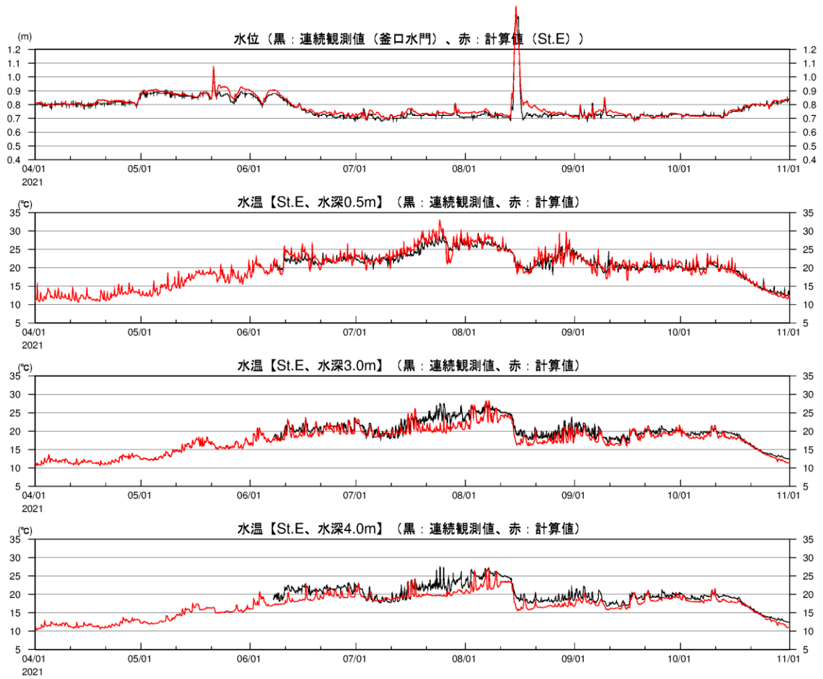
図 2-3(30) 湖内定点の水溫時系列(2021 年、観測結果との比較、St.E)
