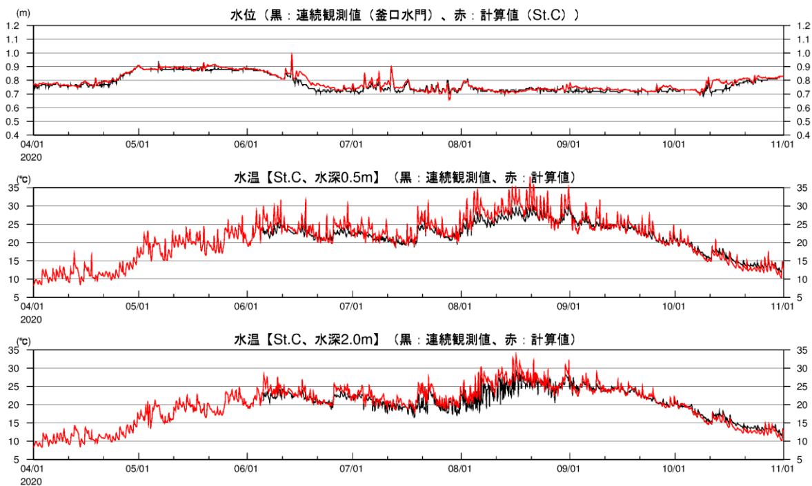
図 2-3(19) 湖内定点の水温時系列(2020年、観測結果との比較、St.C)
