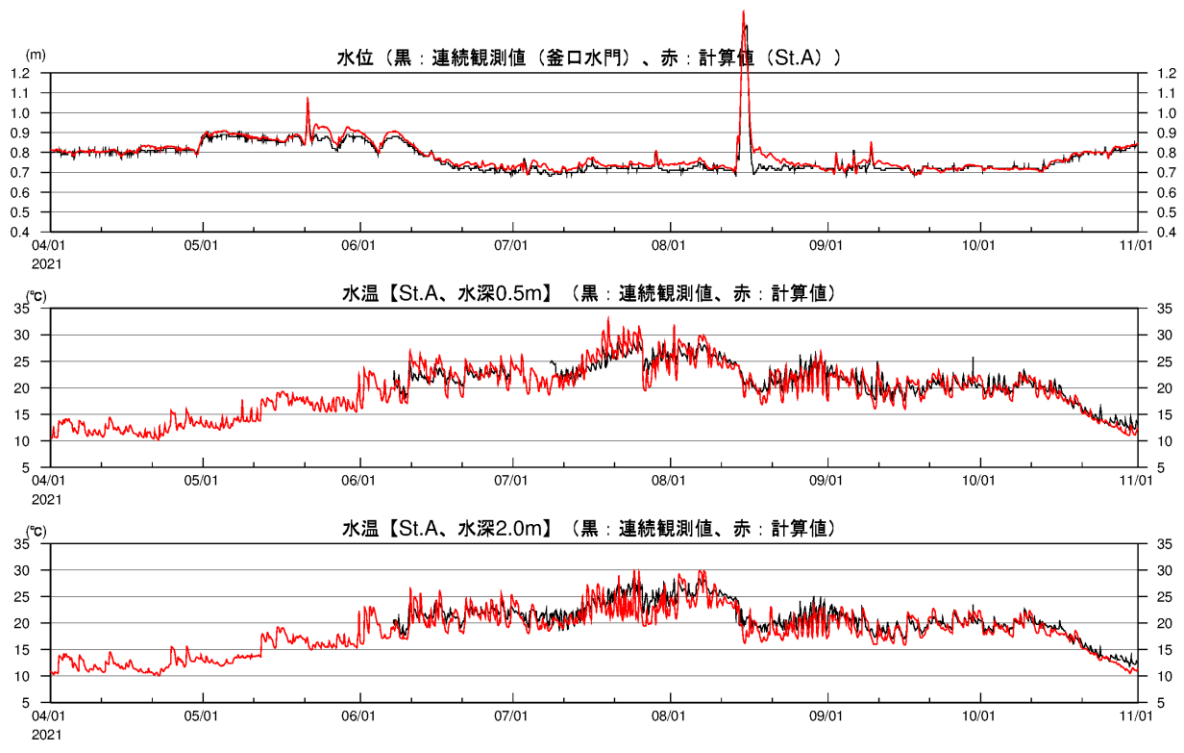
図 2-3(10) 湖内定点の水溫時系列(2021 年、観測結果との比較、St.A)
