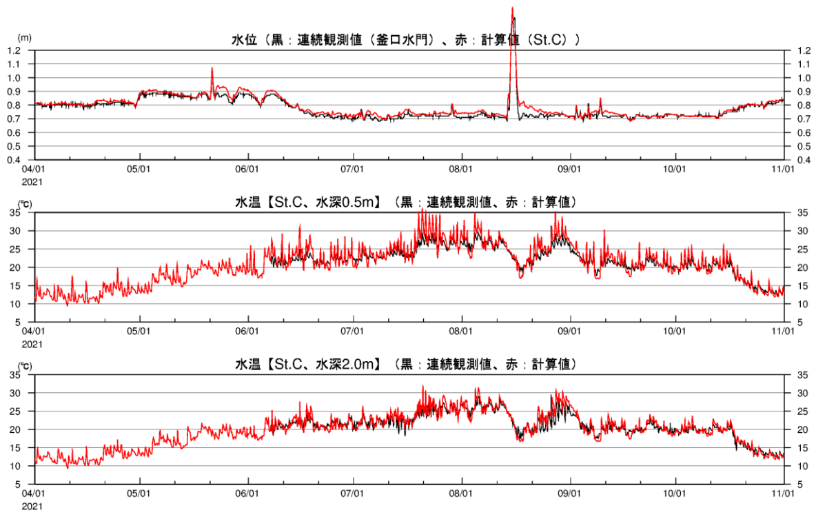
図 2-3(20) 湖内定点の水温時系列(2021 年、観測結果との比較、St.C)
