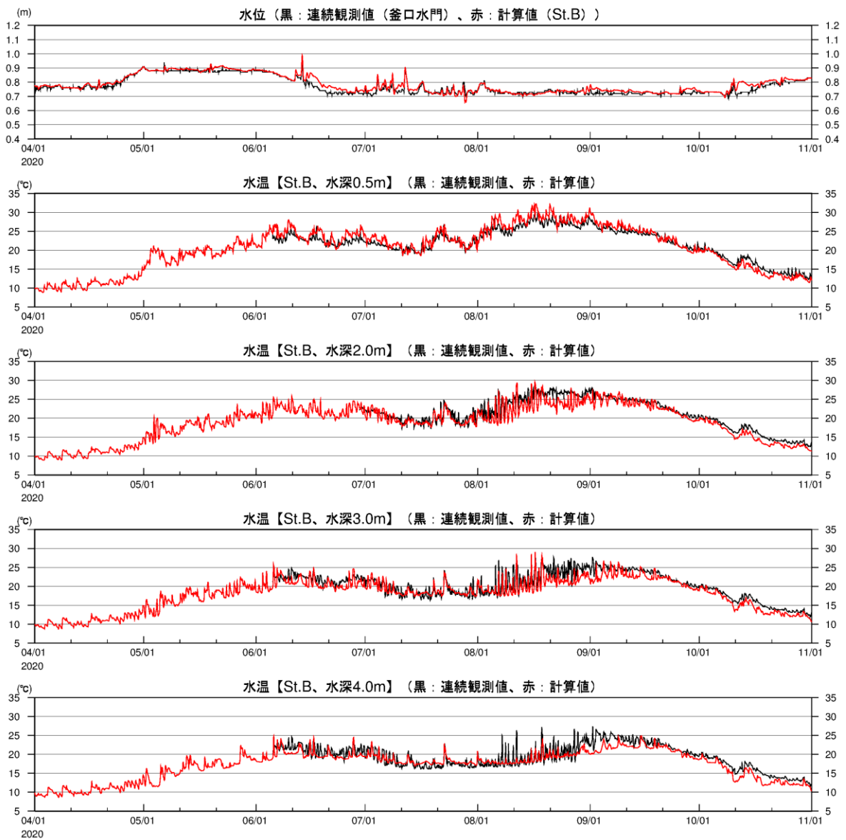
図 2-3(14) 湖内定点の水溫時系列(2020年、観測結果との比較、St.B)
