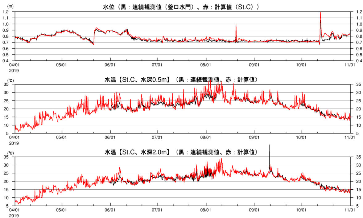
図 2-3(18) 湖内定点の水温時系列(2019年、観測結果との比較、St.C)
