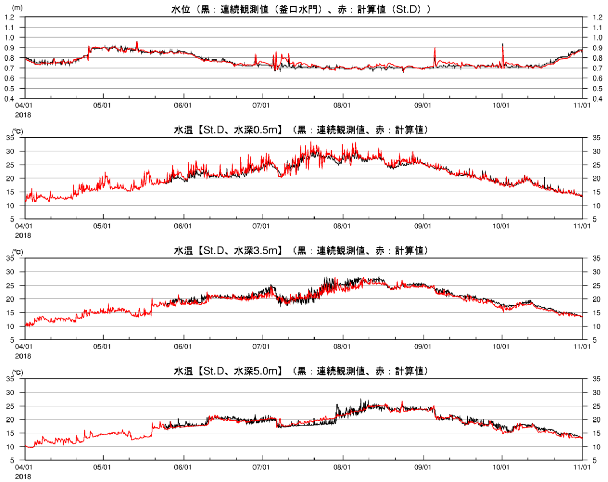
図 2-3(22) 湖内定点の水温時系列(2018年、観測結果との比較、St.D)
