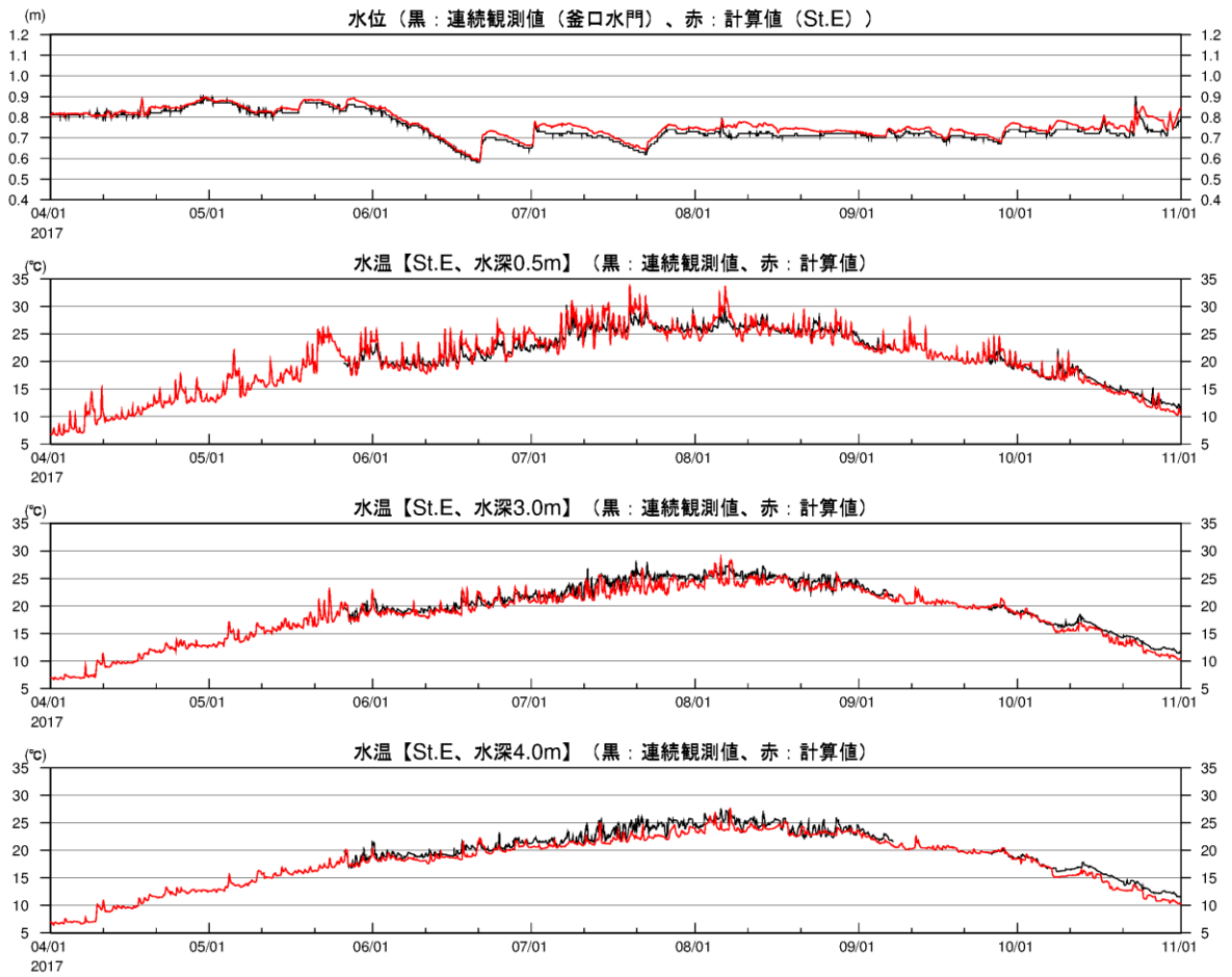
図 2-3(26) 湖内定点の水温時系列(2017年、観測結果との比較、St.E)
