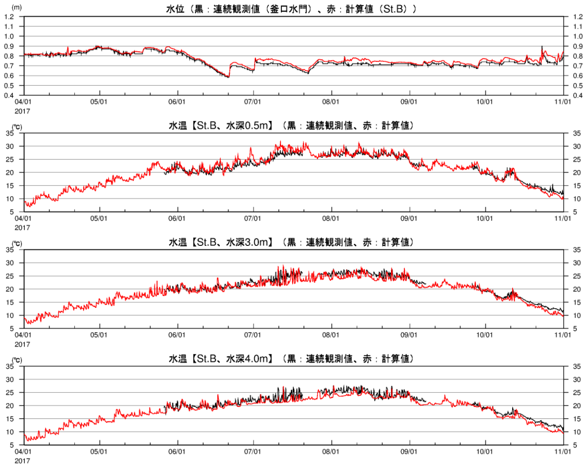
図 2-3(11) 湖内定点の水温時系列(2017年、観測結果との比較、St.B)
