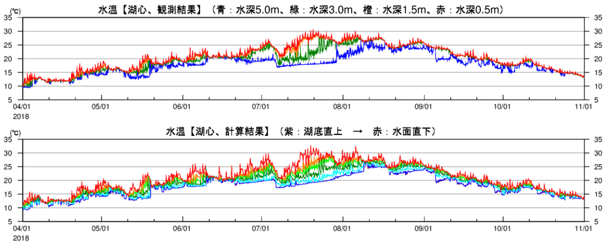
図 2-2(2) 湖心における各水深の水温時系列(2018年、上:観測結果、下:計算結果)
