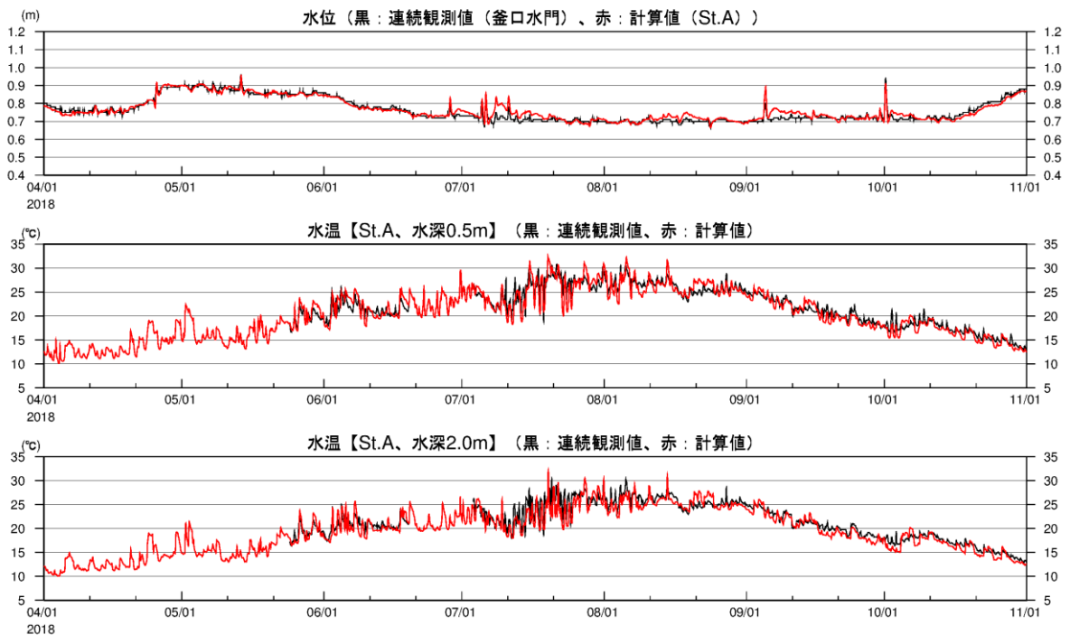
図 2-3(7) 湖内定点の水温時系列(2018年、観測結果との比較、St.A)
