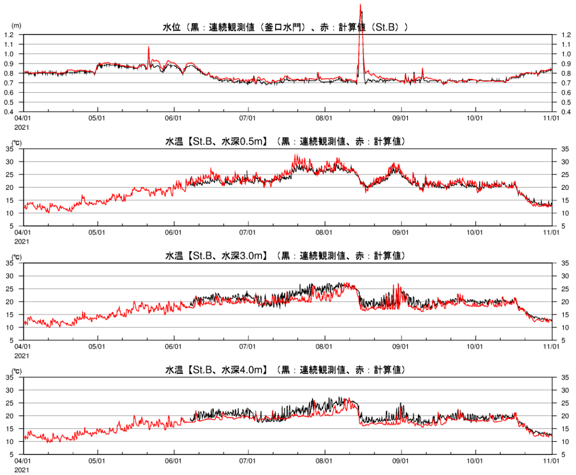
図 2-3(15) 湖内定点の水温時系列(2021年、観測結果との比較、St.B)
