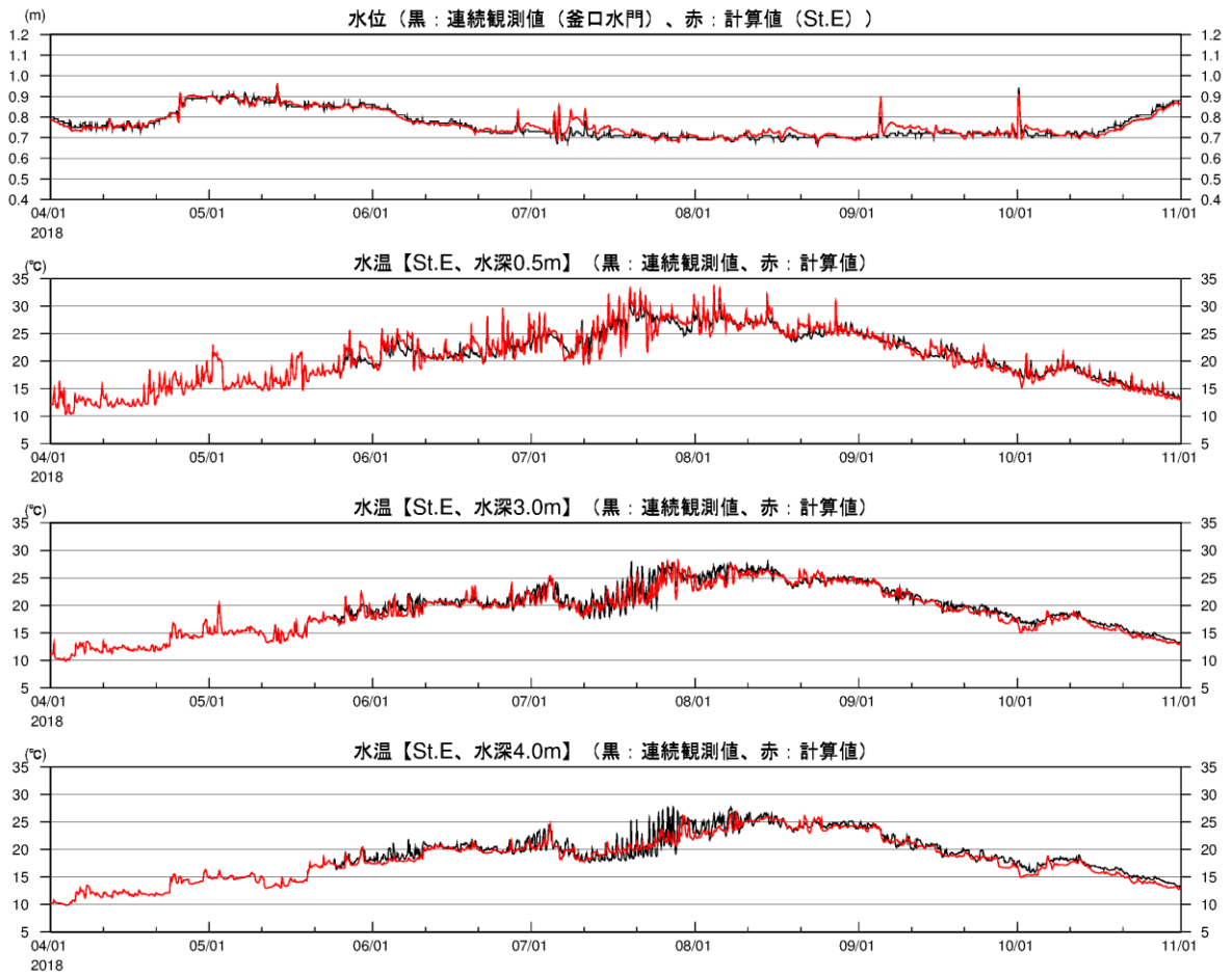
図 2-3(27) 湖内定点の水温時系列(2018年、観測結果との比較、St.E)
