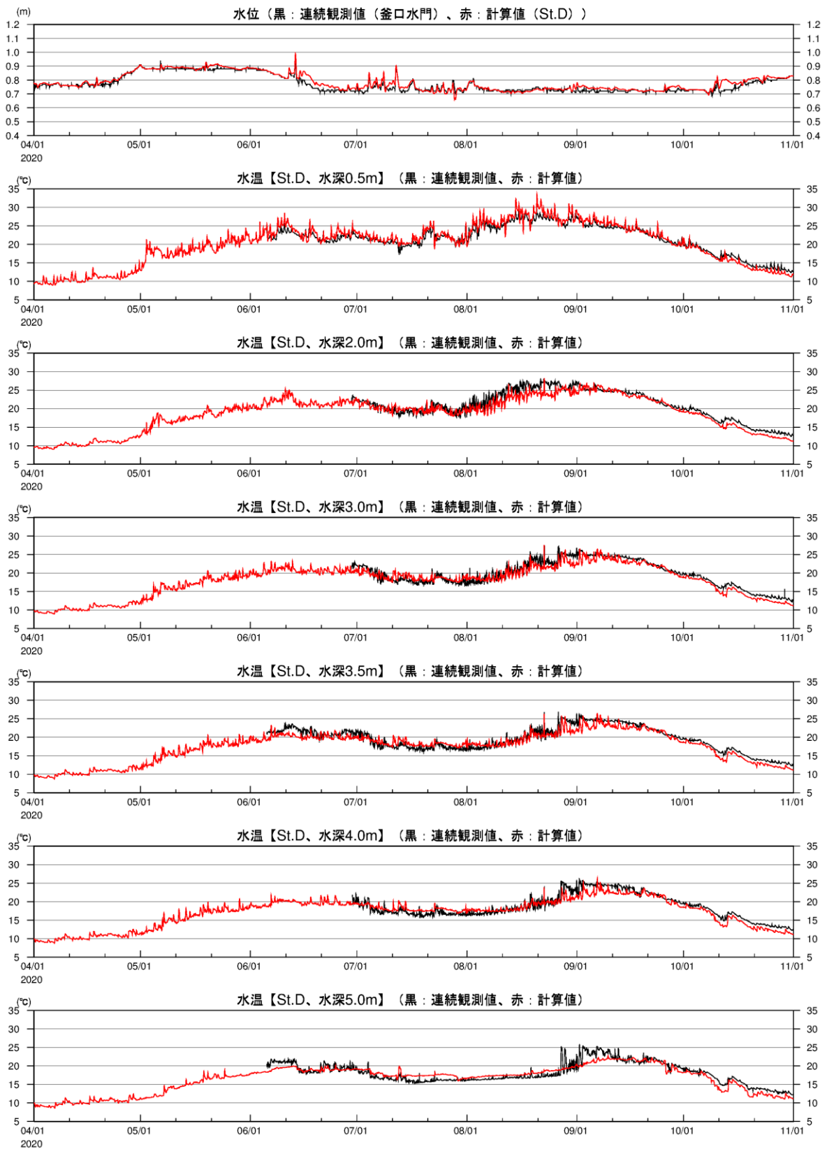
図 2-3(24) 湖内定点の水温時系列(2020年、観測結果との比較、St.D)
