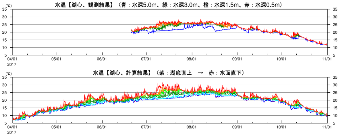
図 2-2(1) 湖心における各水深の水温時系列(2017年、上:観測結果、下:計算結果)
