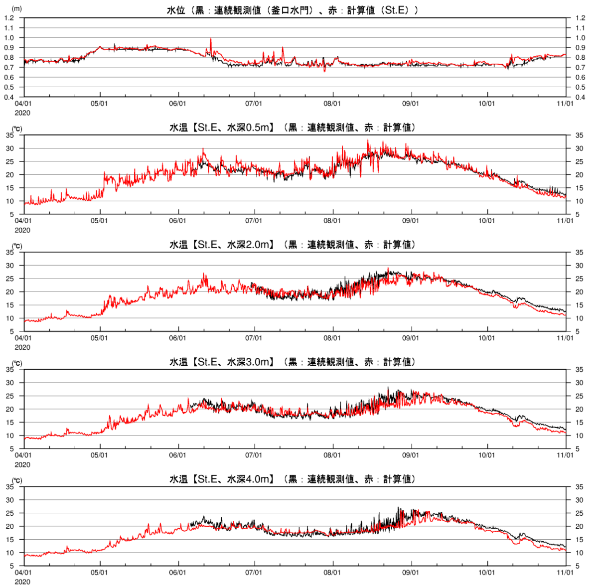
図 2-3(29) 湖内定点の水温時系列(2020年、観測結果との比較、St.E)
