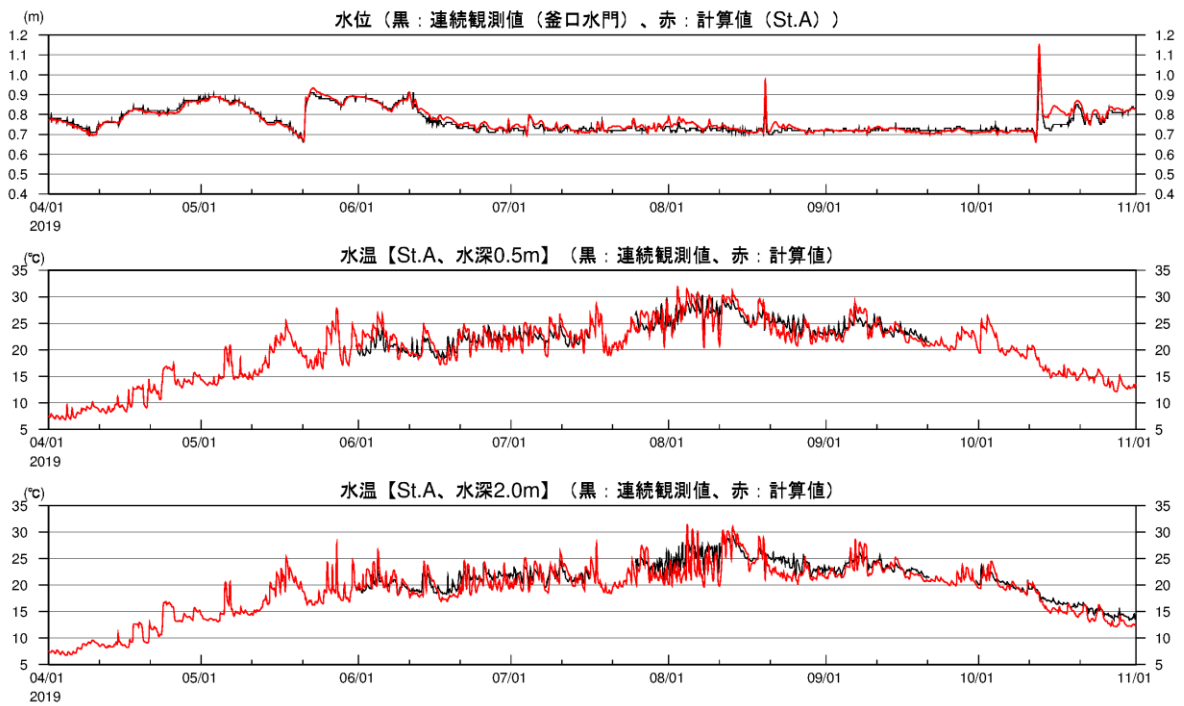
図 2-3(8) 湖内定点の水温時系列 (2019 年、観測結果との比較、St.A)
