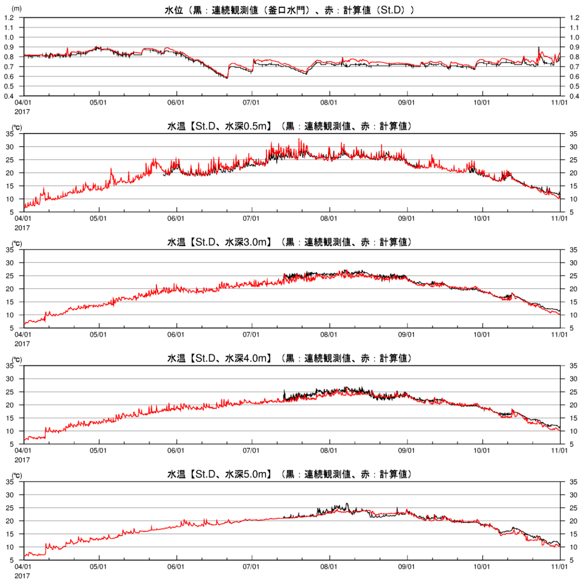
図 2-3(21) 湖内定点の水温時系列(2017年、観測結果との比較、St.D)
