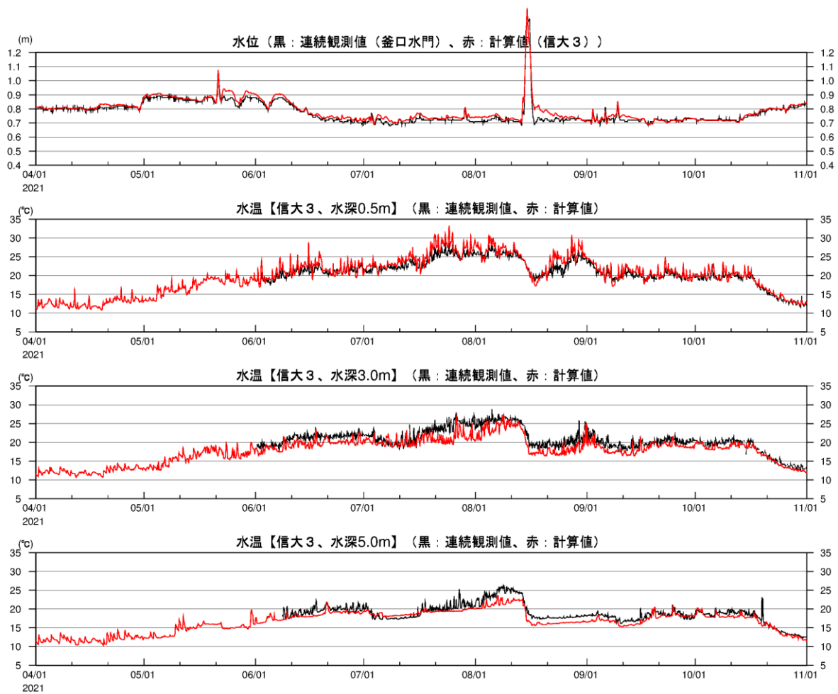
図 2-3(34) 湖内定点の水温時系列(2021年、観測結果との比較、信大③)
