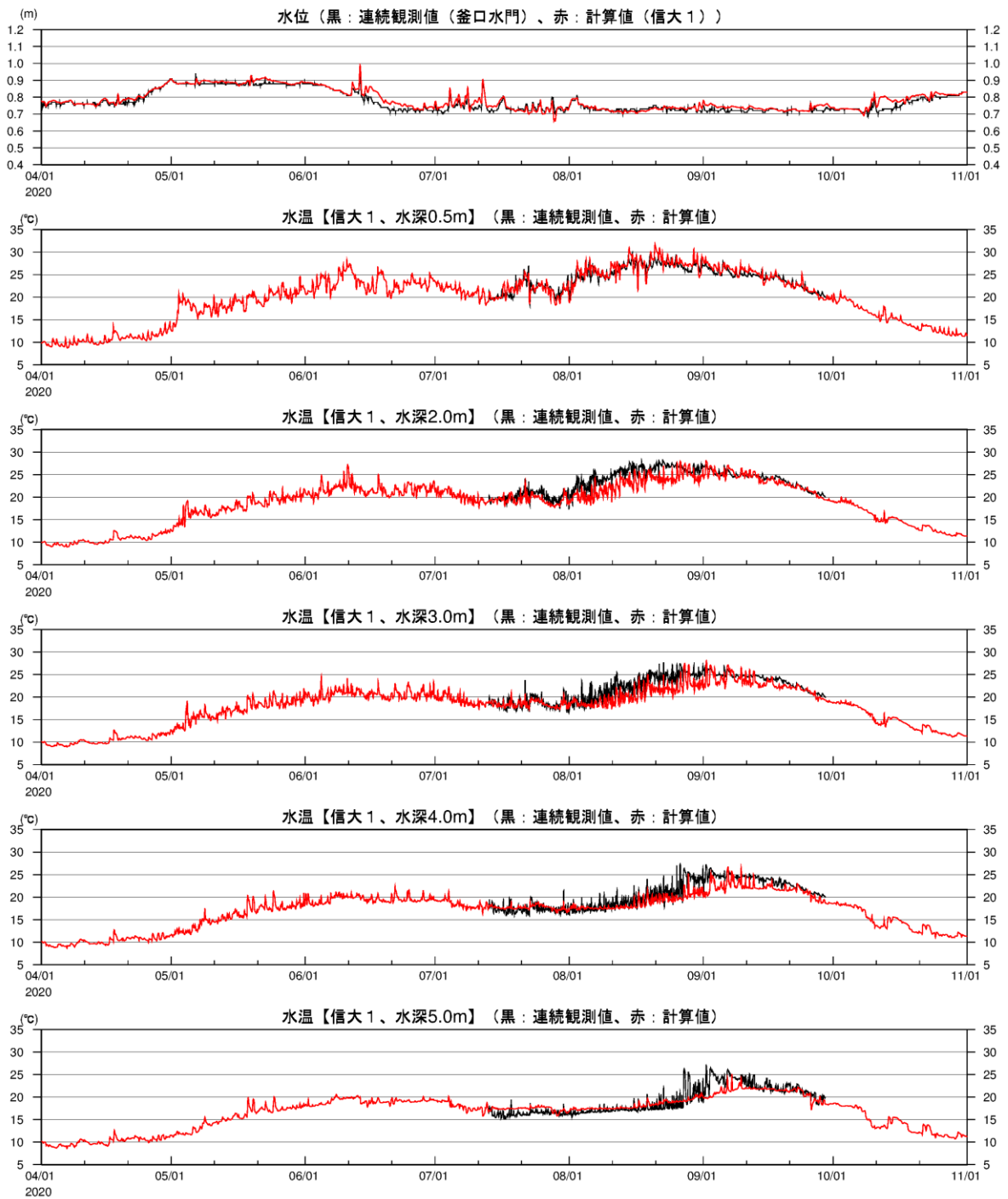
図 2-3(31) 湖内定点の水温時系列(2020年、観測結果との比較、信大①)
