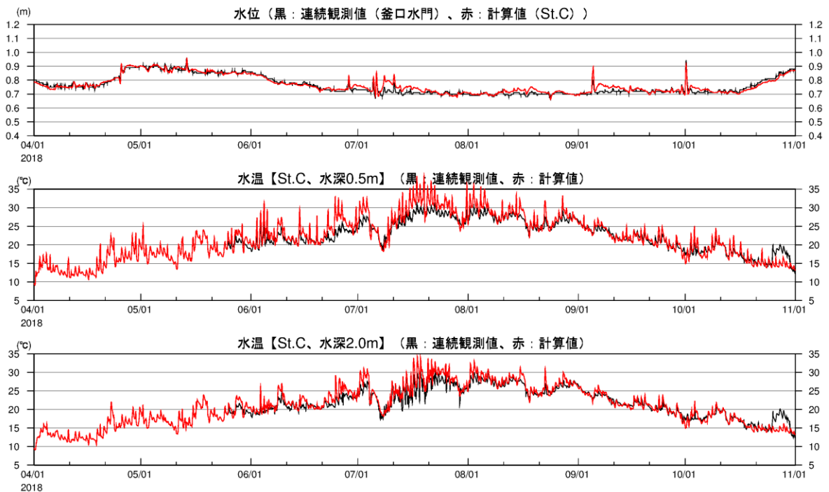
図 2-3(17) 湖内定点の水温時系列(2018年、観測結果との比較、St.C)
