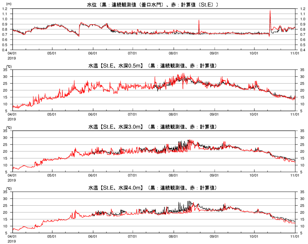
図 2-3(28) 湖内定点の水温時系列(2019年、観測結果との比較、St.E)
