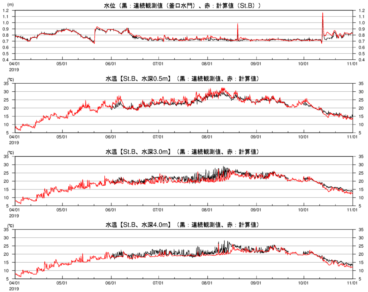
図 2-3(13) 湖内定点の水温時系列(2019年、観測結果との比較、St.B)
