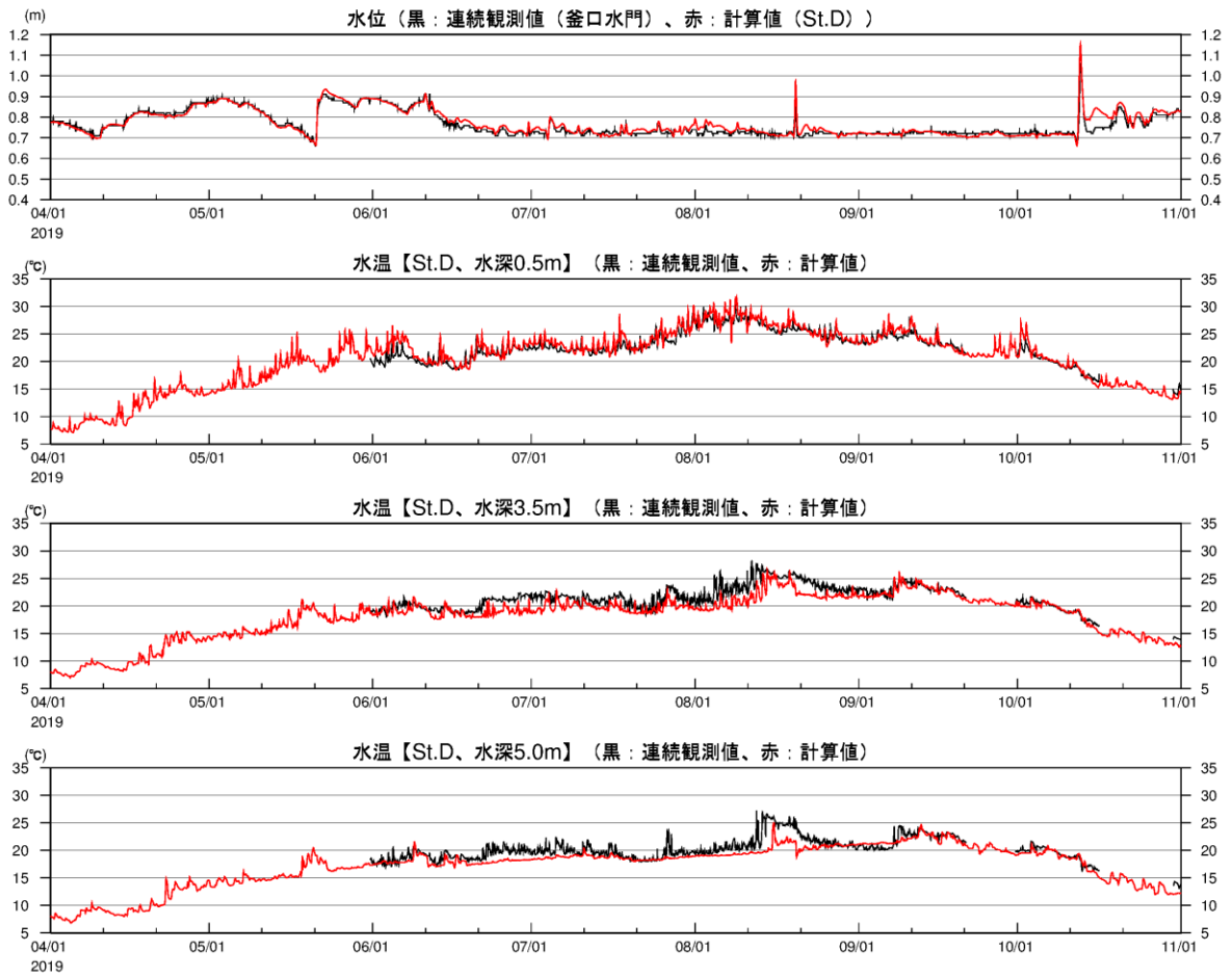
図 2-3(23) 湖内定点の水温時系列(2019年、観測結果との比較、St.D)
