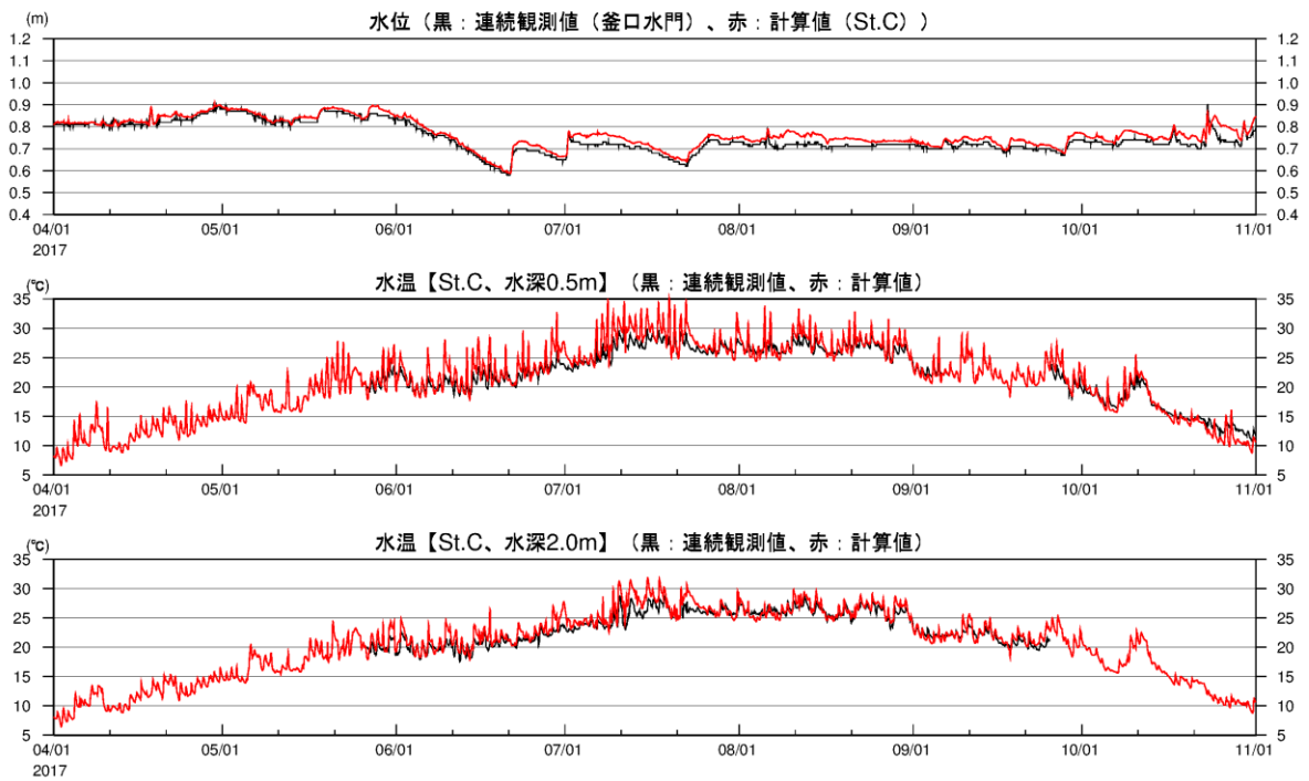
図 2-3(16) 湖内定点の水温時系列(2017年、観測結果との比較、St.C)
