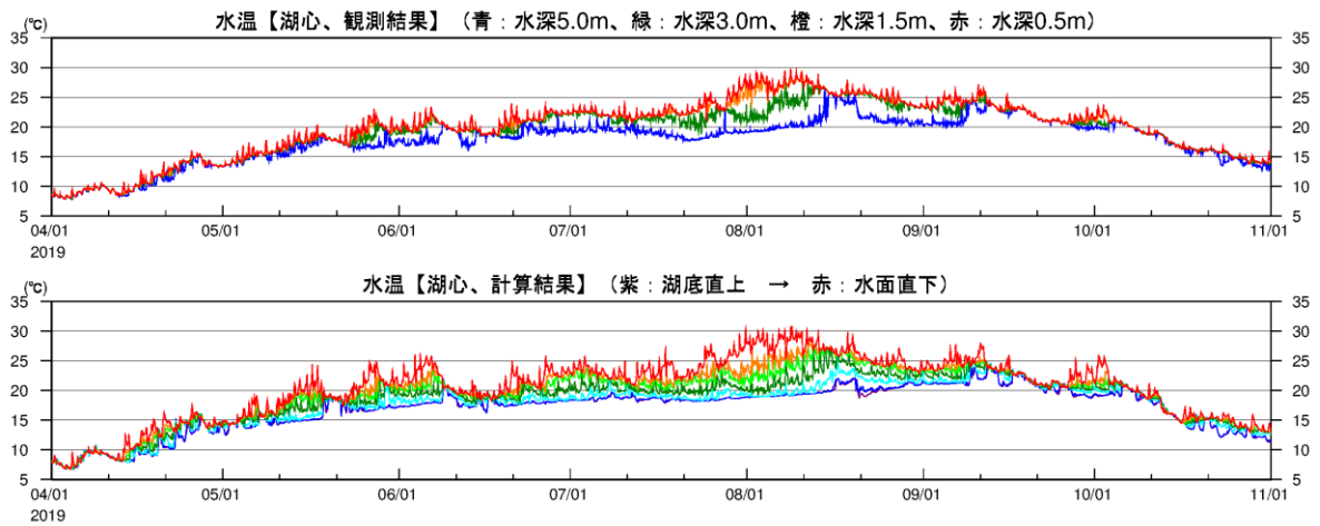
図 2-2(3) 湖心における各水深の水温時系列(2019年、上:観測結果、下:計算結果)
