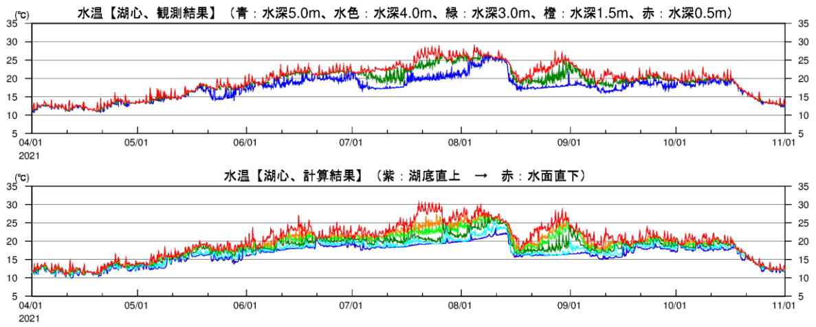
図 2-2(5) 湖心における各水深の水温時系列(2021年、上:観測結果、下:計算結果)
