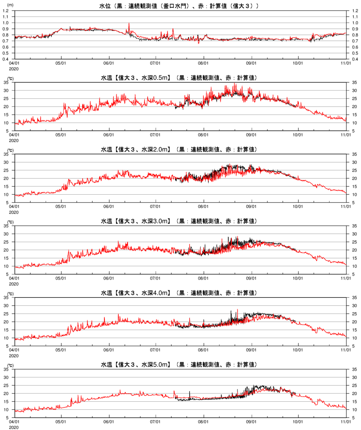
図 2-3(33) 湖内定点の水温時系列(2020年、観測結果との比較、信大③)
