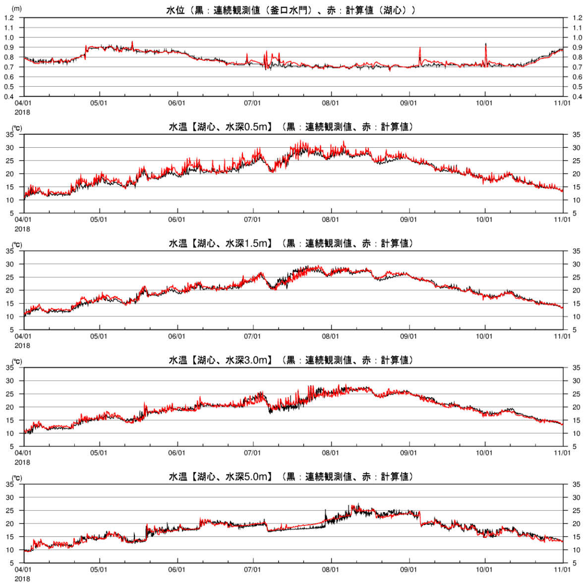
図 2-3(2) 湖内定点の水溫時系列(2018年、観測結果との比較、湖心)
