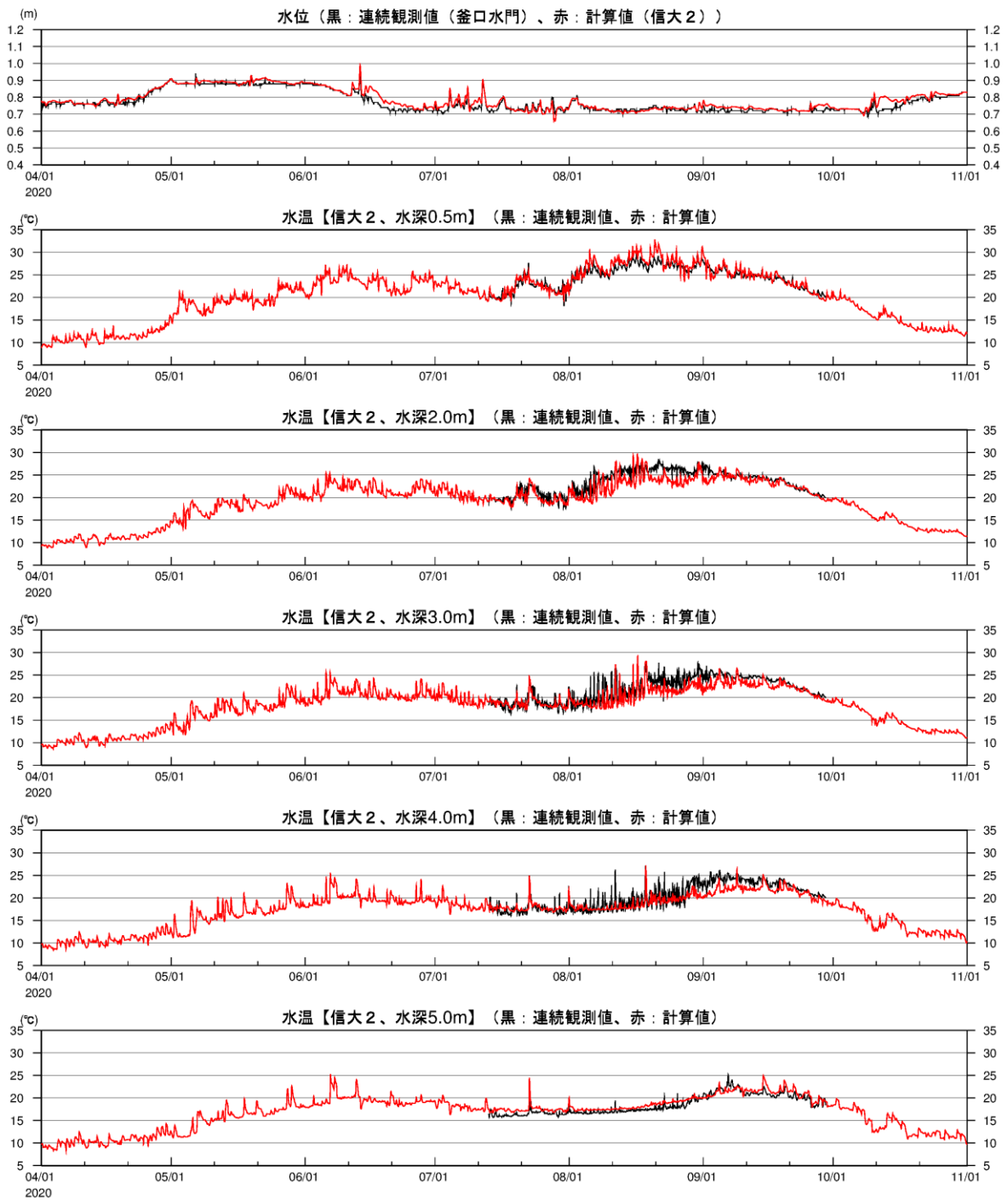
図 2-3(32) 湖内定点の水温時系列(2020年、観測結果との比較、信大②)
