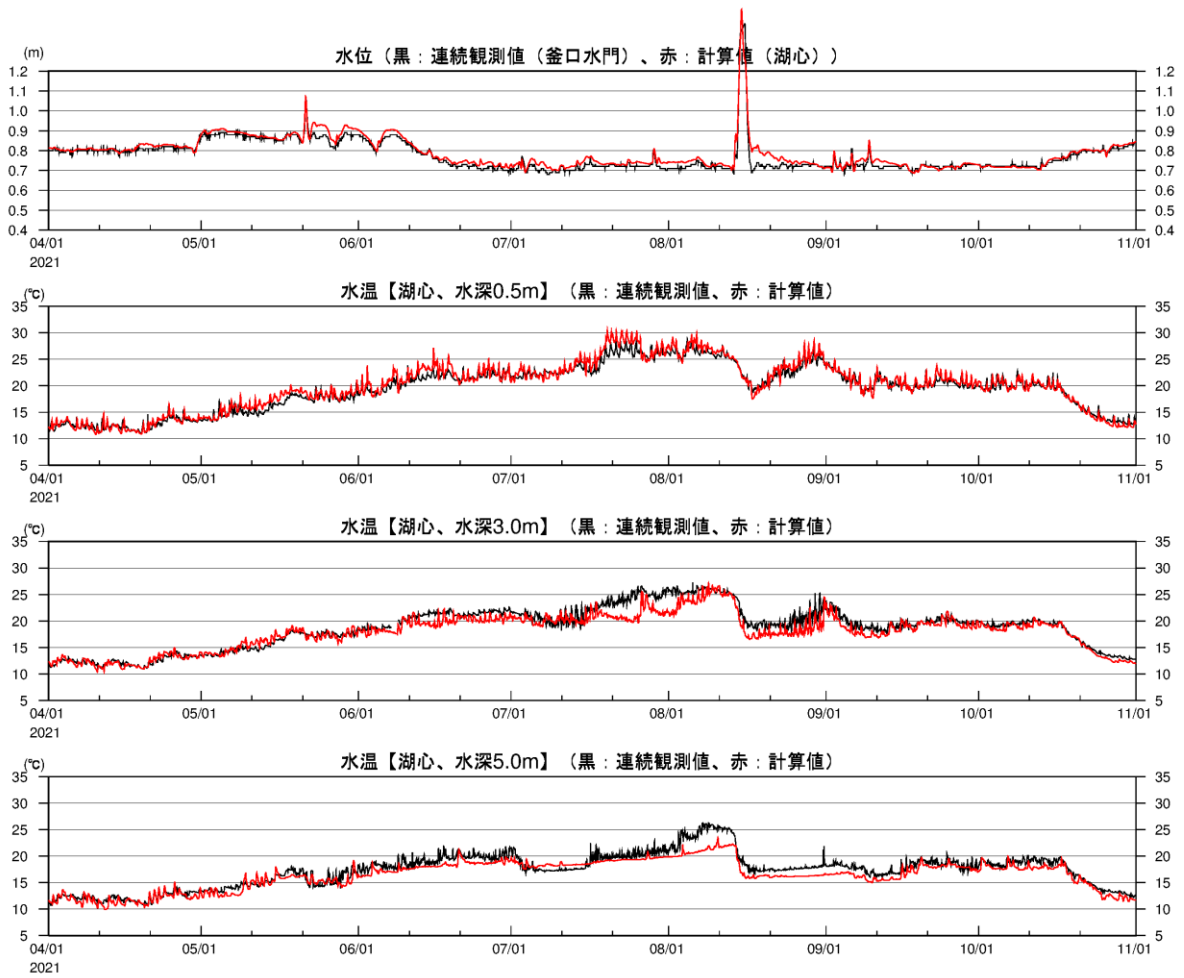
図 2-3(5) 湖内定点の水溫時系列(2021 年、観測結果との比較、湖心)
