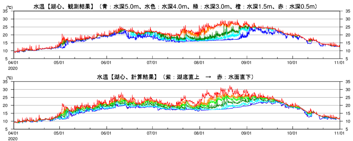
図 2-2(4) 湖心における各水深の水温時系列(2020年、上:観測結果、下:計算結果)
