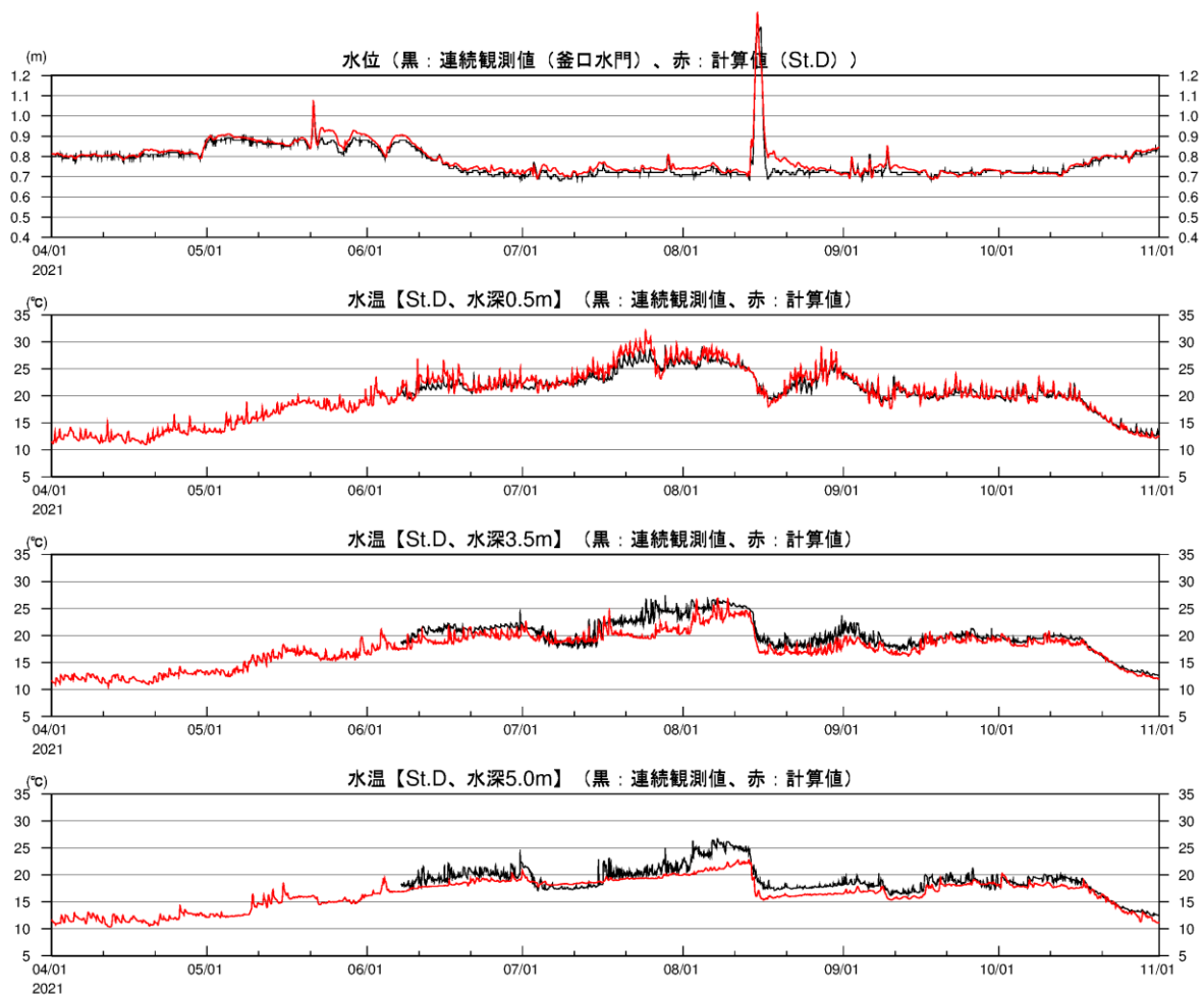
図 2-3(25) 湖内定点の水温時系列(2021年、観測結果との比較、St.D)
