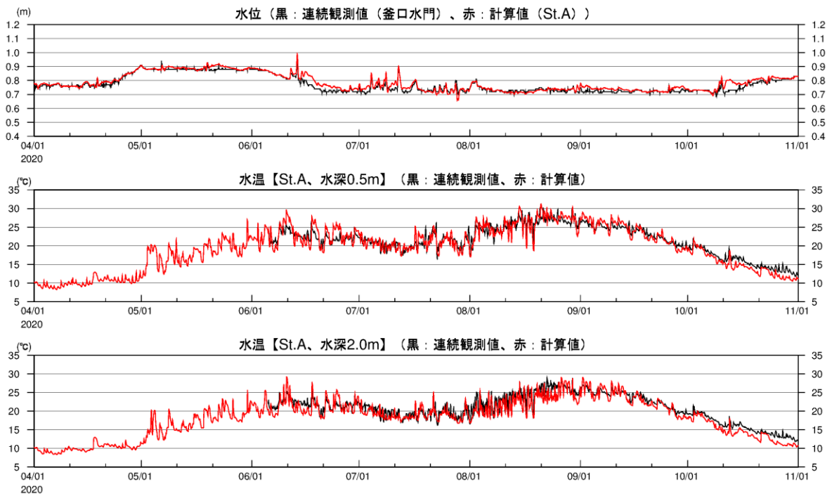
図 2-3(9) 湖内定点の水温時系列 (2020 年、観測結果との比較、St.A)
