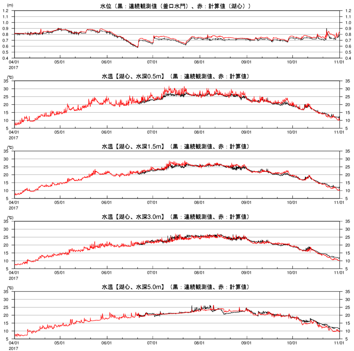
図 2-3(1) 湖内定点の水温時系列(2017年、観測結果との比較、湖心)
