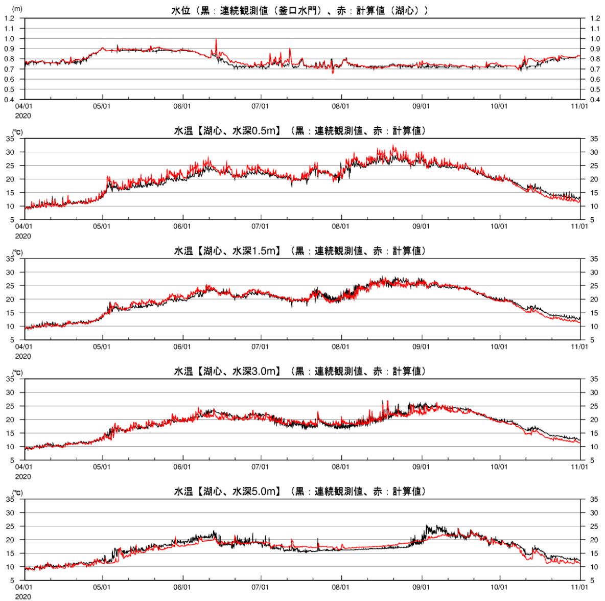
図 2-3(4) 湖内定点の水溫時系列(2020年、観測結果との比較、湖心)
