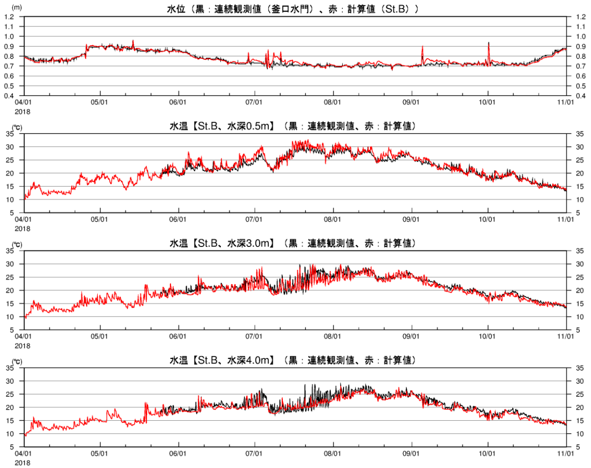
図 2-3(12) 湖内定点の水温時系列(2018年、観測結果との比較、St.B)
