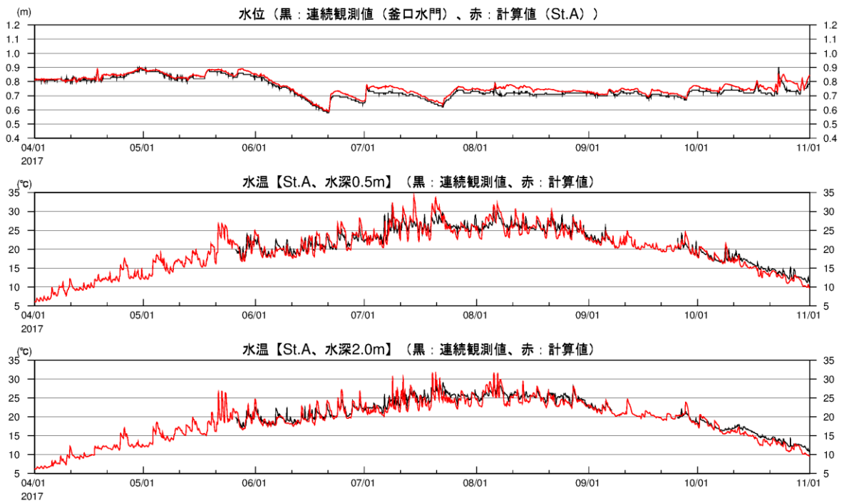
図 2-3(6) 湖内定点の水温時系列(2017年、観測結果との比較、St.A)
