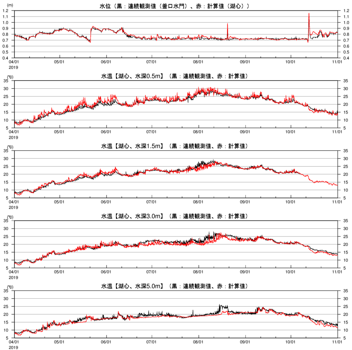
図 2-3(3) 湖内定点の水温時系列(2019年、観測結果との比較、湖心)
