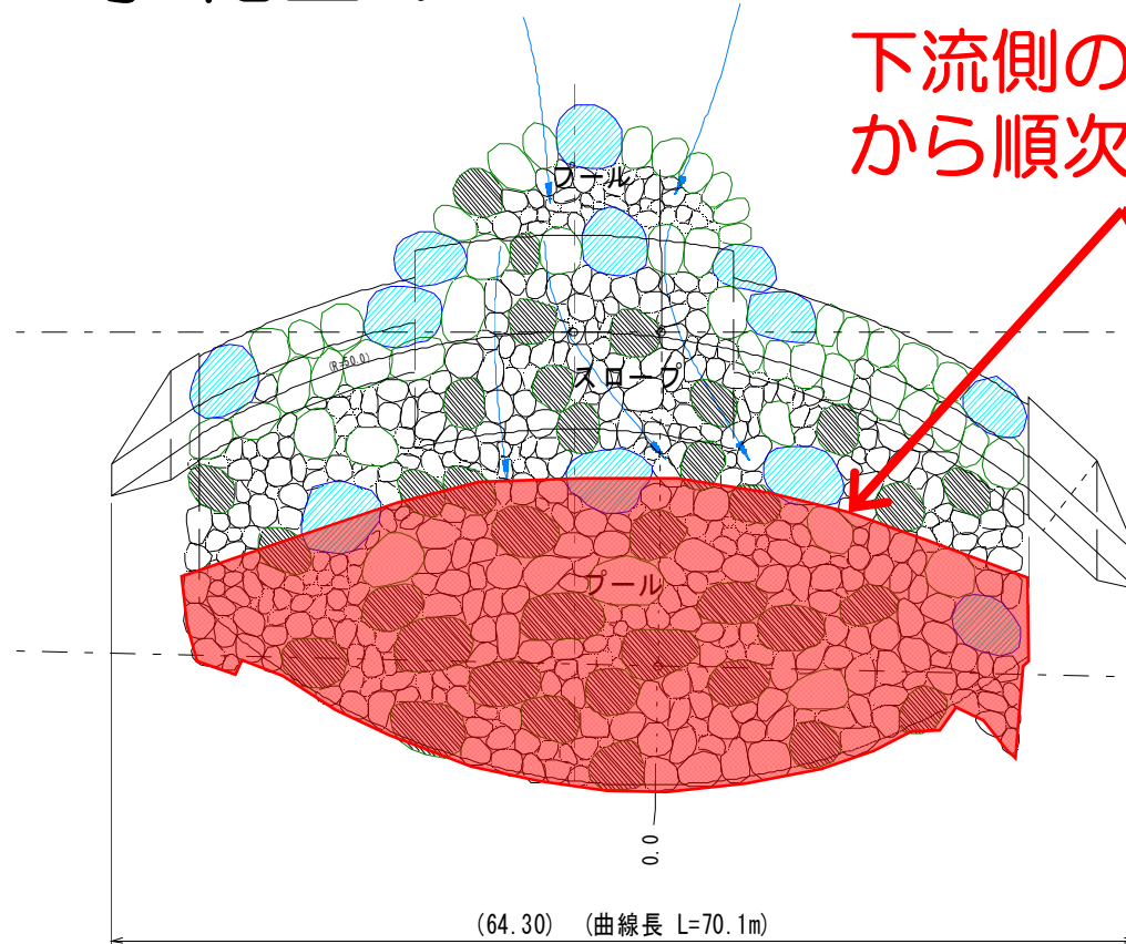
帯工構造図
