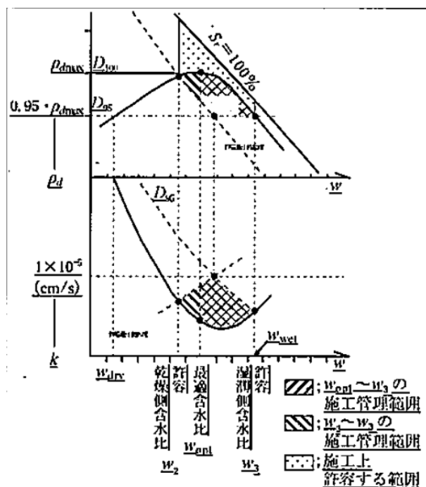
図-4.3.2 築堤材料の施工管理範囲の例
