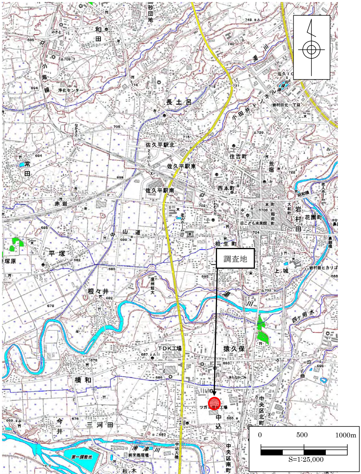
図 4-1-1 調査位置図 縮尺 1 : 25,000 国土地理院数値地図より
