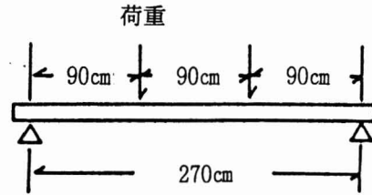
図-1 実大材曲げ試験条件
