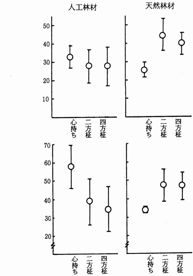
図-11 正角の木取り別、最大節径比、集中節径比の平均値と標準偏差
