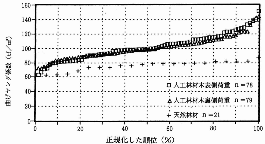
図-16 人工林正角（荷重方向別）と天然林正角実大材の正規化した曲げヤング係数の分布
