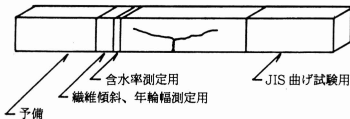
図-3 実大材曲げ試験終了材から各試験体の採材
