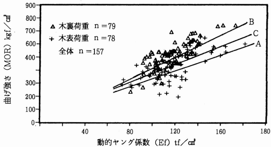
図-18 人工林カラマツ正角の実大材曲げ破壊試験における動的ヤング係数 (Ef) と曲げ強さ (MOR) の関係
