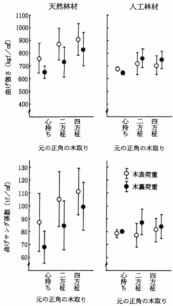
図-14 JIS曲げ試験における曲げ強さ、曲げヤング係数の平均値、標準偏差
