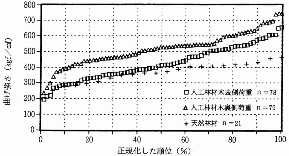
図-15 人工林正角（荷重方向別）と天然林正角実大材の正規化した曲げ強さの分布
