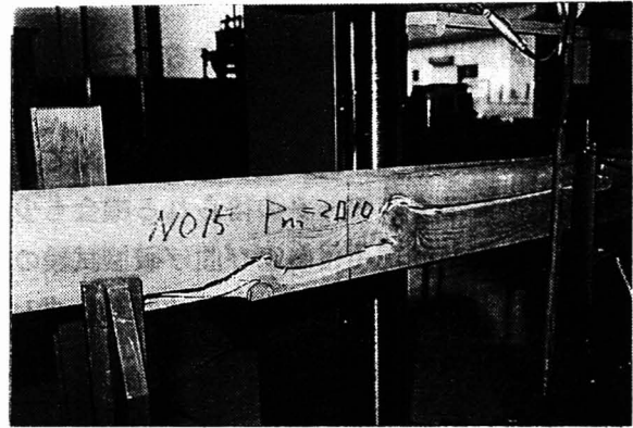
写真-3 節の撮影が認められる破壊例
