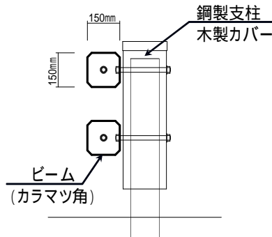
図-2 2号型の構造図
