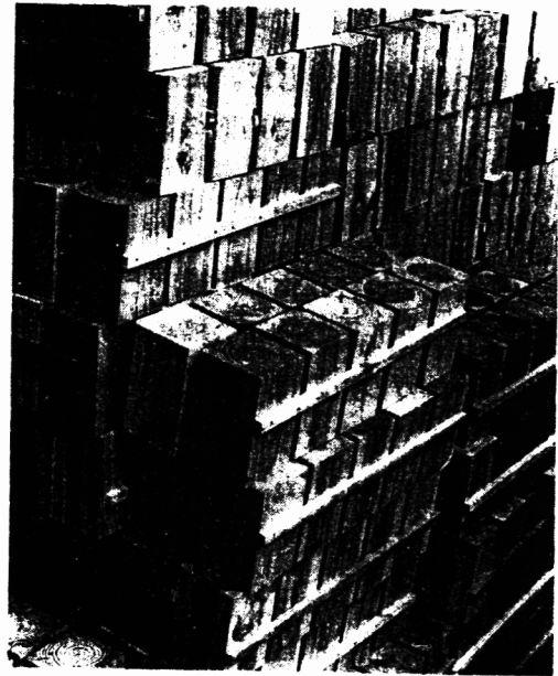
写真-3 完成した木レンガユニット
