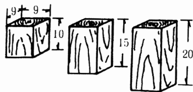
木レンガブロック
