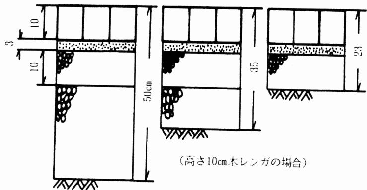
図-3 基礎部分を変えた木レンガ歩道断面図
