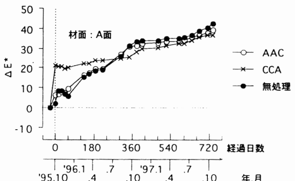
図6-9 色差の経時変化（A面）
