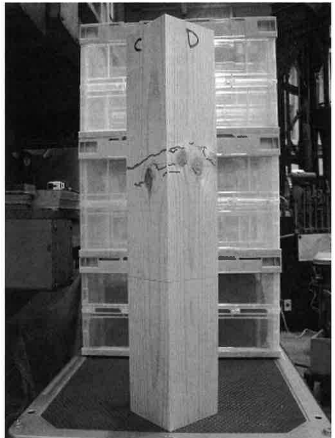
写真-5 アカマツグループC (高温乾燥材) 試験後
