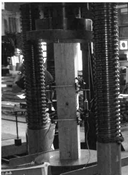
写真-1 圧縮試験の状況
