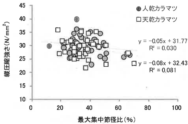
図-10 カラマツの最大集中節径比と縦圧縮強さ
