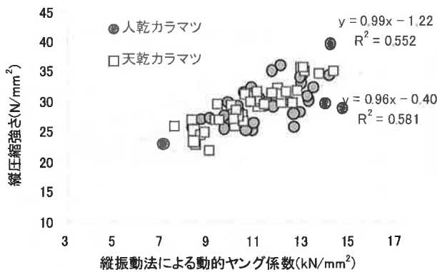
図-14 カラマツの動的ヤング係数と縦圧縮強さ
