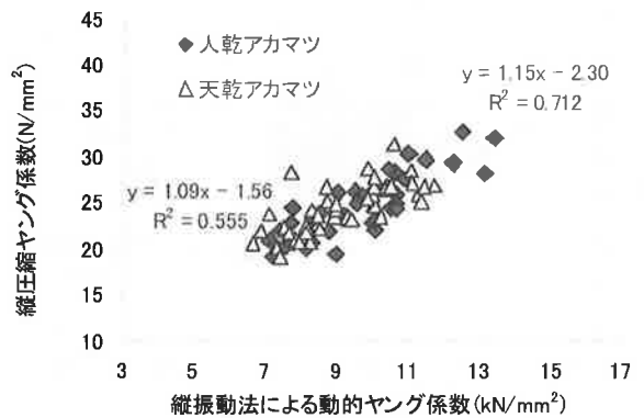
図-15 アカマツの動的ヤング係数と縦圧縮強さ
