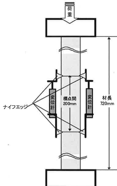
図-1 試験体と変位計の設置方法
