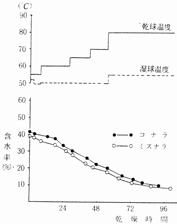
図一 1 コナラ ミズナラ 30mm人工乾燥含水率経過図 (24時間連続運転)
