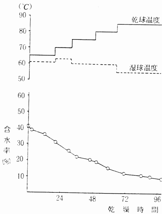
図一 2 ニセアカシア 30mm人工乾燥含水率経過図 (24時間連続運転)
