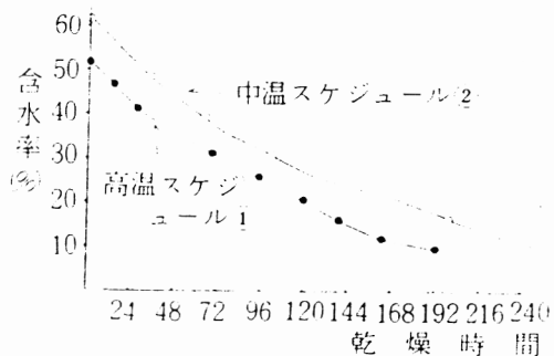
図-5 ミズナラ36mm人工乾燥含水率経過図 (12時間間欠運転)
