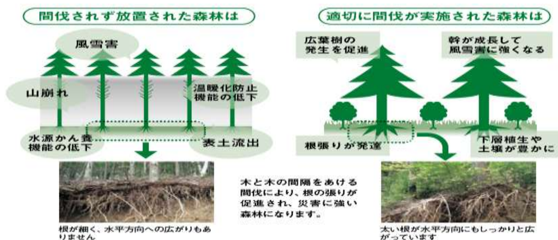
図4 間伐の効果
