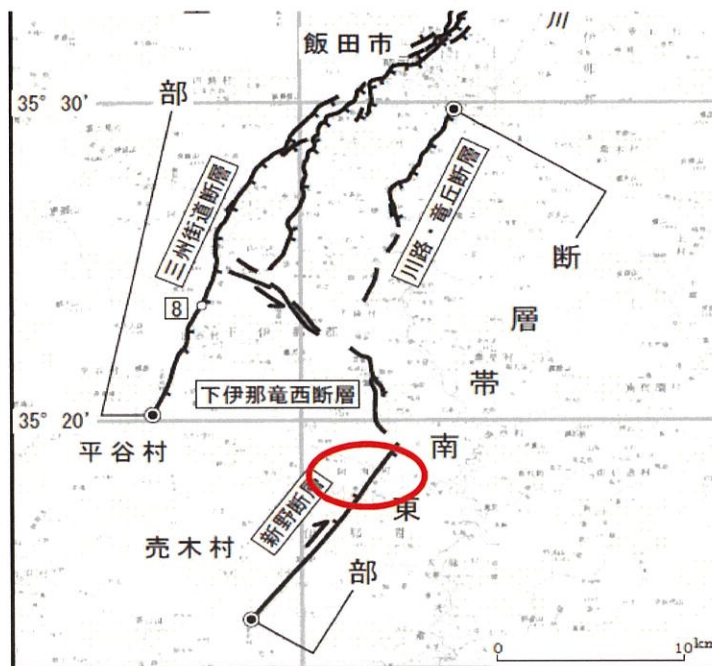
図2 伊那谷断層帯南東部（新野断層）の位置
