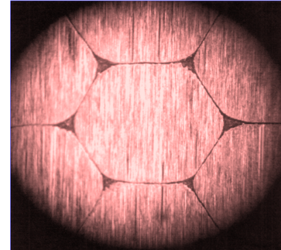
占積率97%のコイル断面写真
