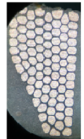
圧縮成型後
