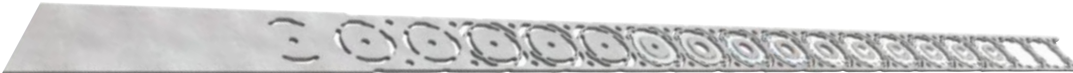
超精密冷間鍛造順送プレス工法の工程レイアウト
