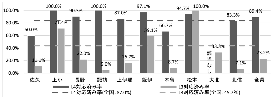
図6-14 クリプトスポリジウム対策済み施設率
