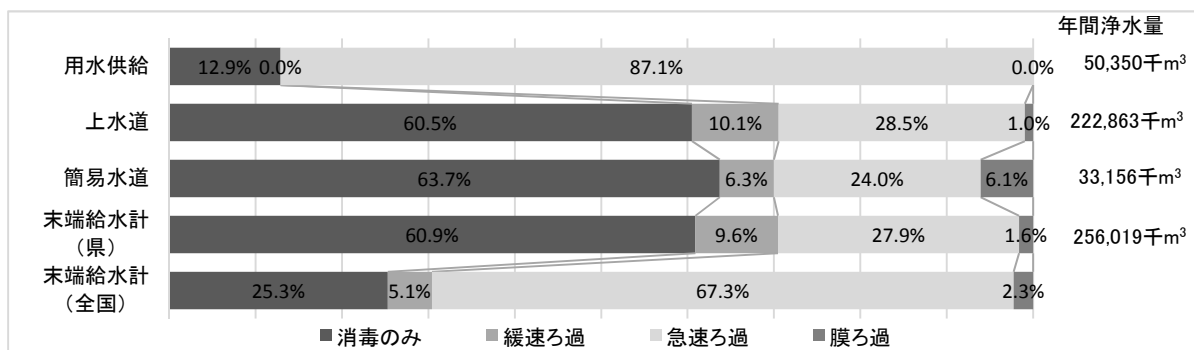
図3-8 浄水方法の構成(平成26年度)
