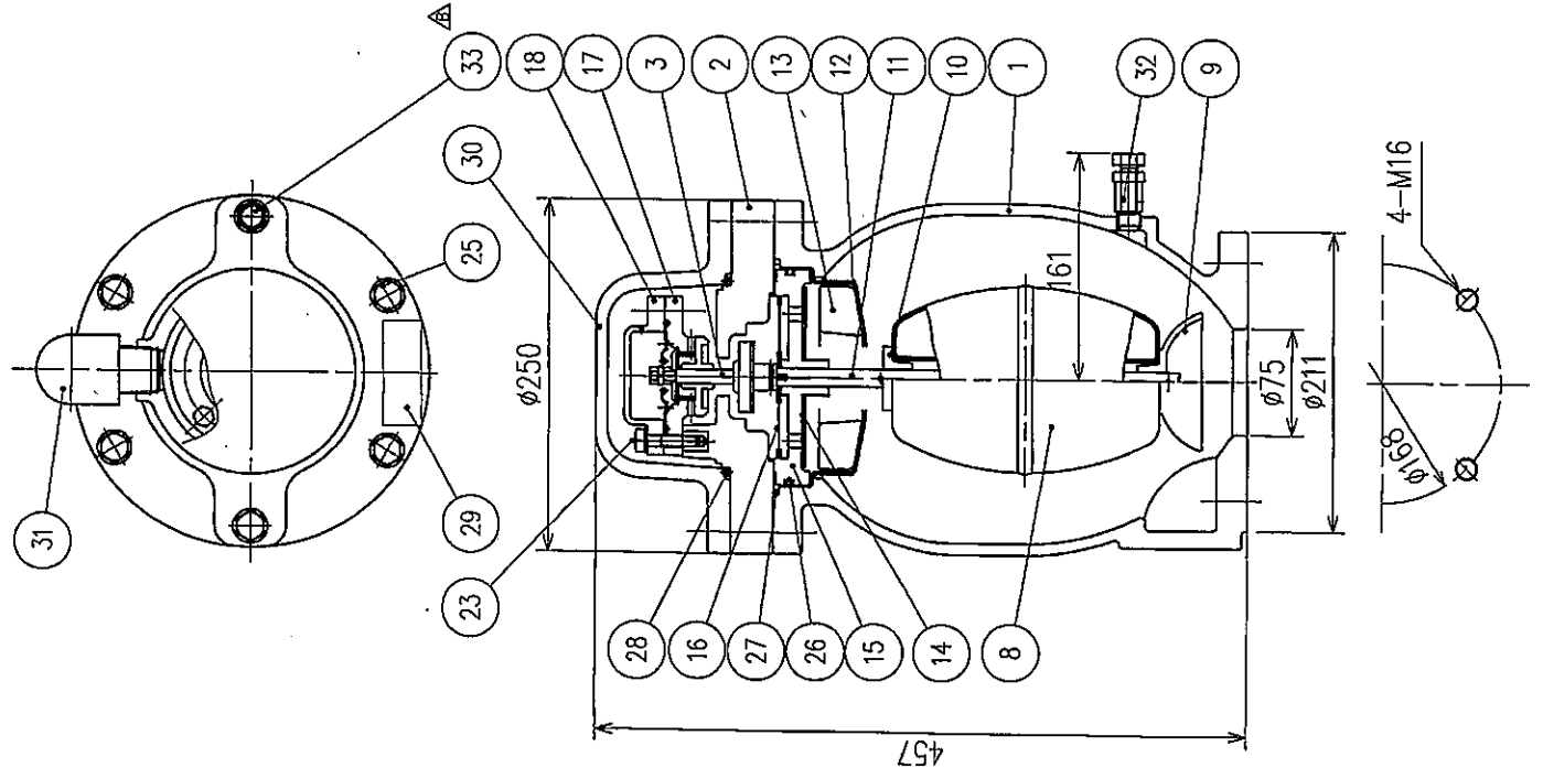
圧力室、弁座部詳細(1/2)
