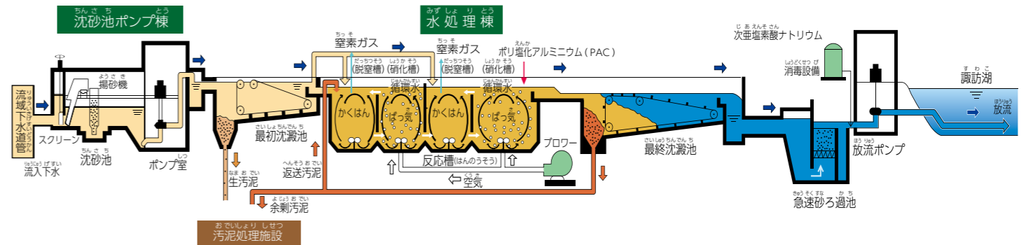
クリーンレイク諏訪(豊田終末処理場)の水処理施設の仕組み
